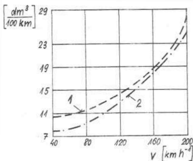
Obr. 4.2 Závislost spotřeby na rychlosti vozidla [1]
