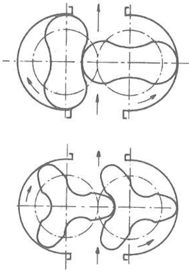
Obr. 2.2 Průřezy rotorů Rootsova dmyhadla [1]
