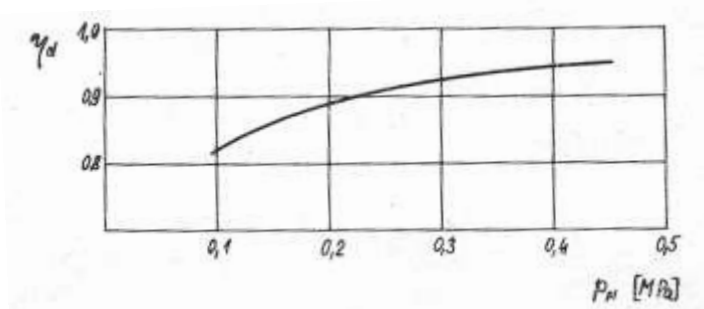
Obr. 1.2 Závislost dopravní účinnosti na plnicím tlaku [1]
