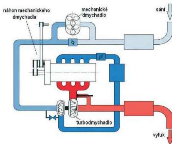
Obr. 7.5 Přeplňování typu Twincharger [3]
