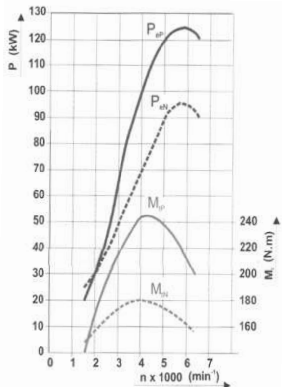
Obr. 1.1 Porovnání výkonů a točivých momentů [2]
