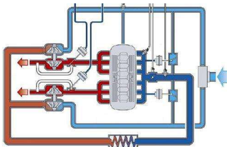
Obr. 7.4 Paralelní Twin-Turbo [17]
