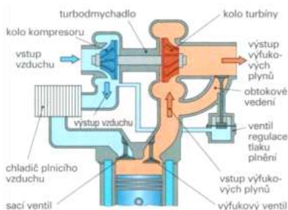
Obr. 3.4 Obtékání spalin za turbínu [12]
