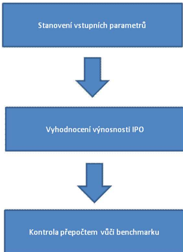
Obrázek 21: Algoritmus výpočtu
