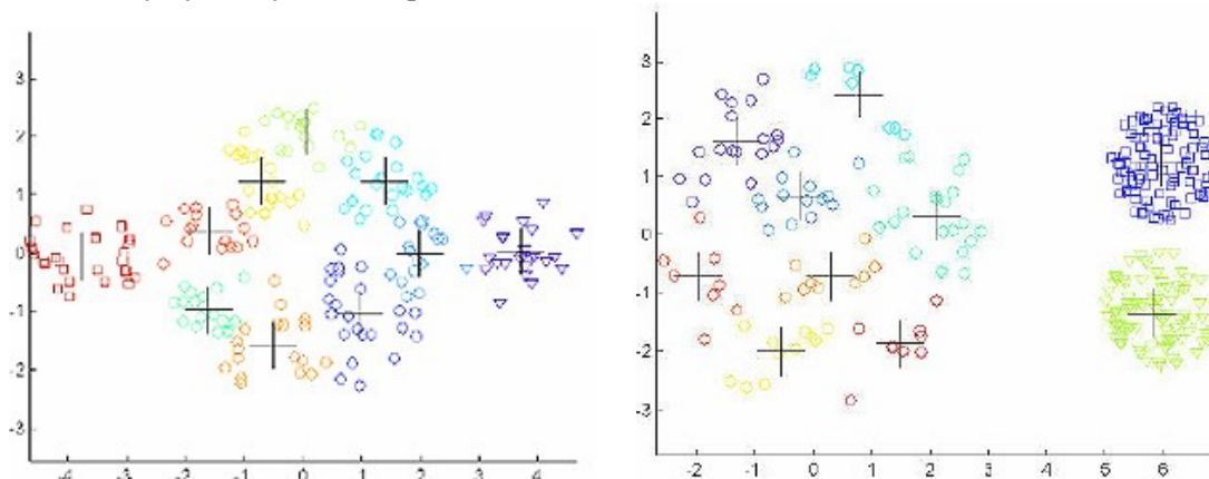
Obrázek 2.8: Použití většího počtu shluků pro zamezení promíchání dat z různých tříd [4]
