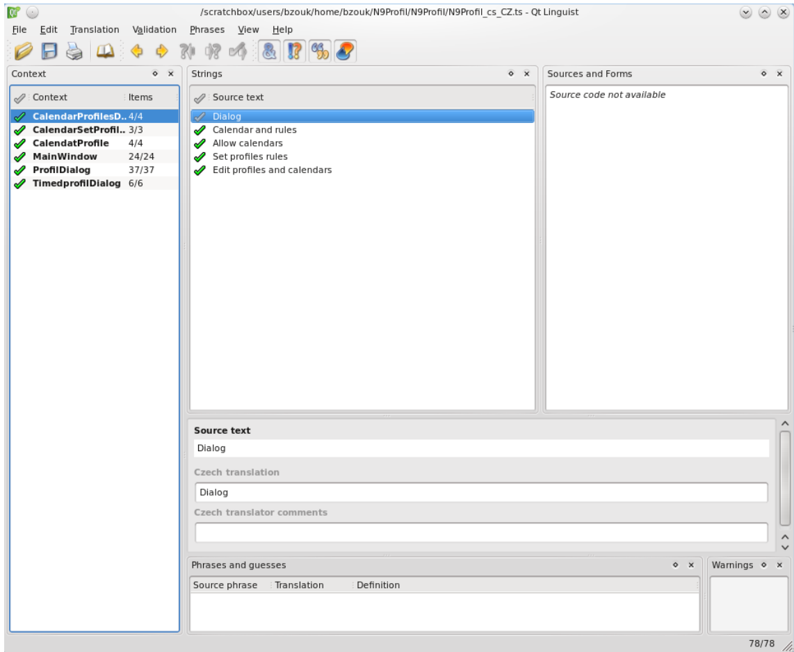
Obrázek 2.8: Qt Linguist
