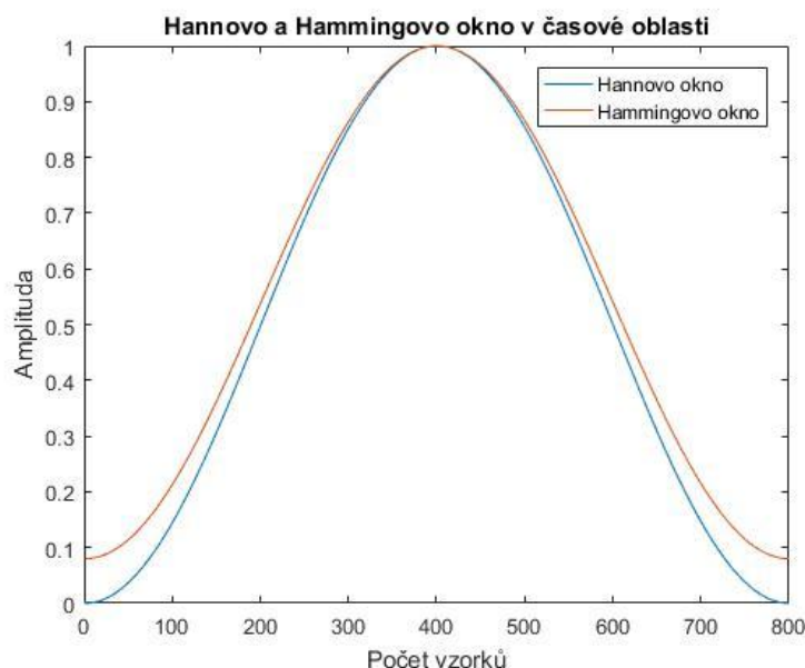
Obr. 2.1: Srovnání Hannova a Hammingova okna.
