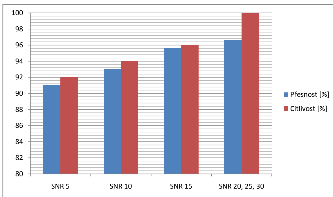
Obr. 6.3: Prvotní testování metody podpůrných vektorů pro lineární funkci.
