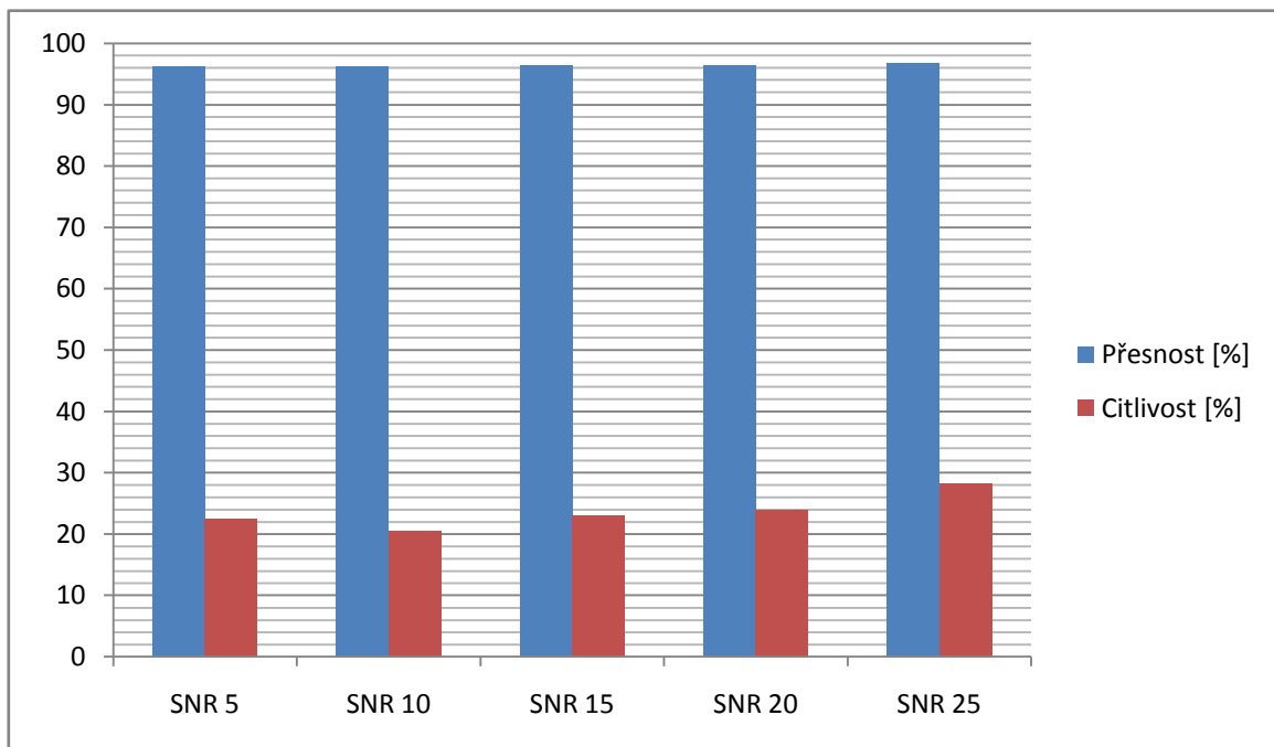
Obr. 8.4: Metoda TotalBoost pro 100 rozhodovacích stromů při různých hodnotách SNR.
