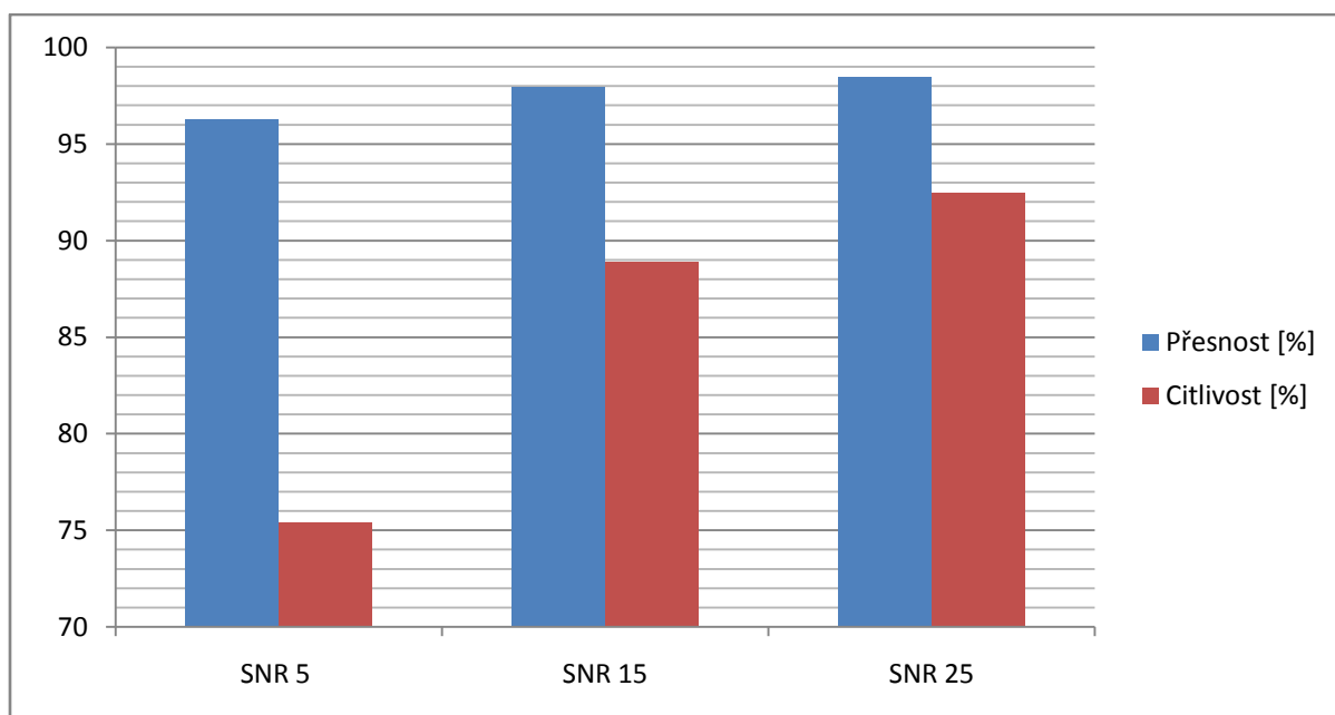
Obr. 9.1: Metoda TotalBoost pro 100 trénovacích stromů při využití statistických veličin.
