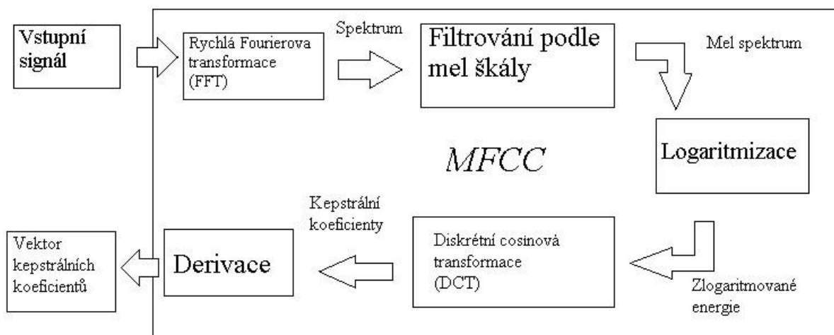
Obr. 3.1: Standardní blokové schéma systému Melovských kepstrálních koeficientů.
