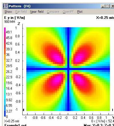
Obr. 24 Srovnání rozložení složky E_y intenzity elektrického pole na rovinné ploše
