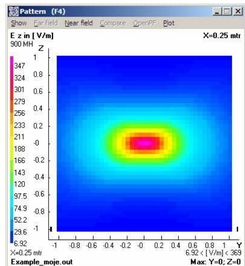
Obr. 29 Srovnání rozložení složky E_z intenzity elektrického pole na rovinné ploše
