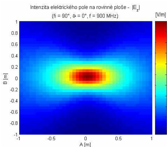
Obr. 25 Srovnání rozložení složky E_z intenzity elektrického pole na rovinné ploše
