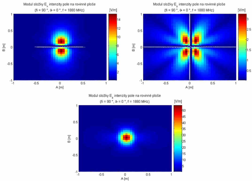
Obr. 42 Rozložení kartézských složek intenzity elektrického pole antény F-Panel na rovinné ploše
