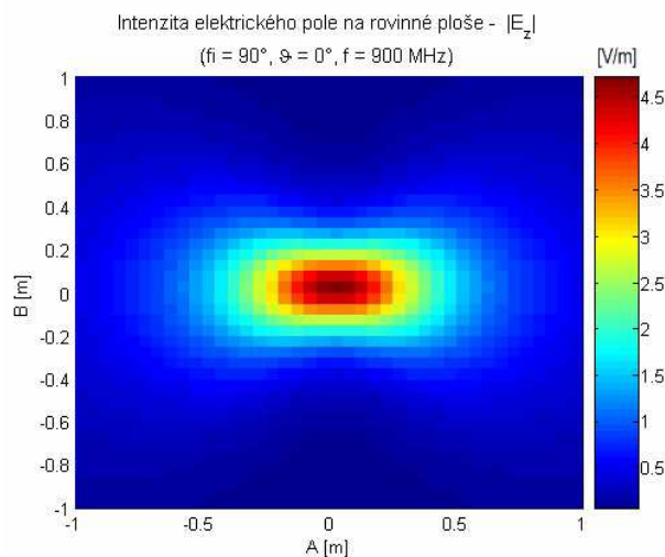
Obr. 29 Srovnání rozložení složky E_z intenzity elektrického pole na rovinné ploše
