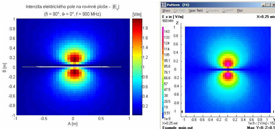
Obr. 27 Srovnání rozložení složky E_x intenzity elektrického pole na rovinné ploše
