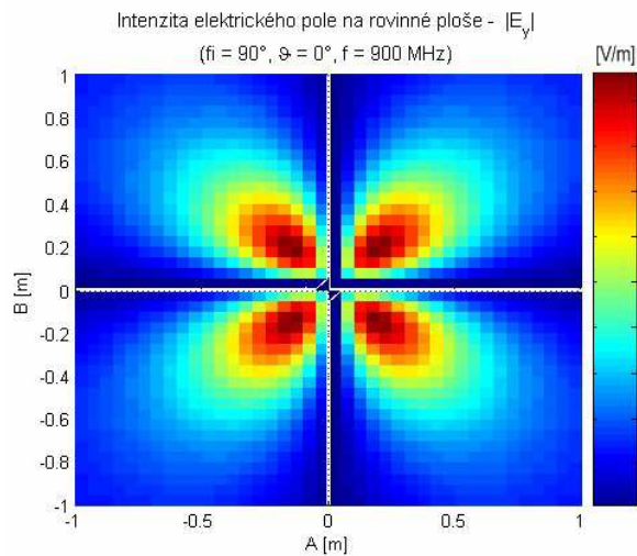
Obr. 28 Srovnání rozložení složky E_y intenzity elektrického pole na rovinné ploše
