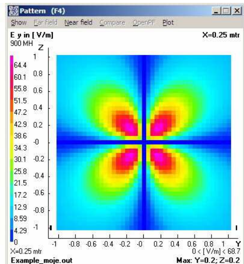
Obr. 28 Srovnání rozložení složky E_y intenzity elektrického pole na rovinné ploše
