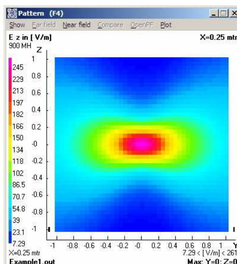
Obr. 25 Srovnání rozložení složky E_z intenzity elektrického pole na rovinné ploše
