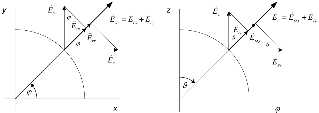
Obr. 13 Sférické souřadnice – výpočet složky \vec{E}_r
