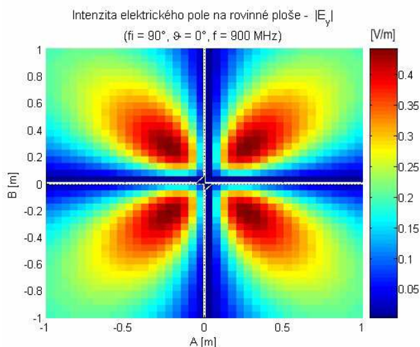
Obr. 24 Srovnání rozložení složky E_y intenzity elektrického pole na rovinné ploše
