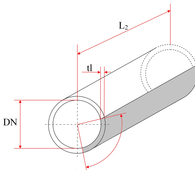
Obr. 2.5: Rozmery rúrky pre výrez lopatky podľa [7]
