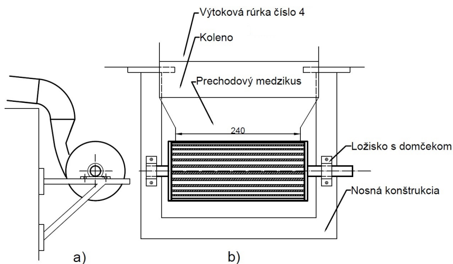
Obr. 4.14: Znáznornenie uchytenia turbíny
