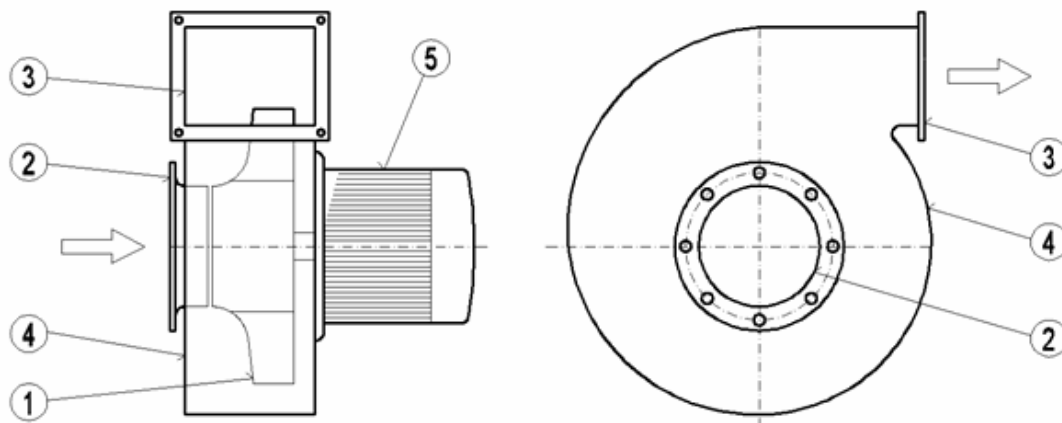
Obr. 1.2 — Radiální ventilátor [5]
