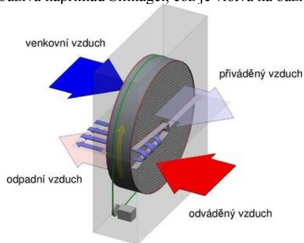
Obr. 1.7 — Rotační regenerační výměník [10]
