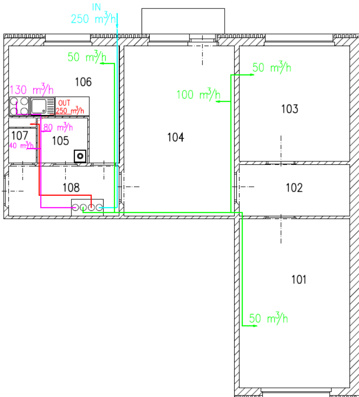
Obr. 3.1 — Schéma potrubní sítě pro jednotku Futura L
