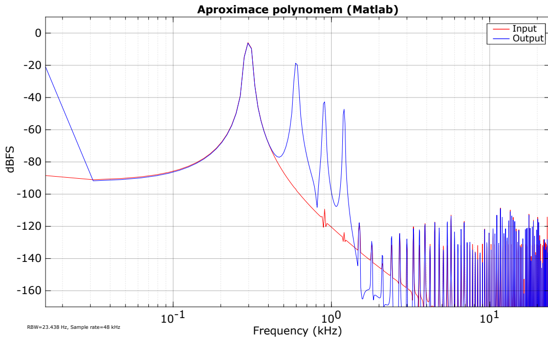
Obr. 3.7: Kmitočtové spektrum výstupního signálu po zkraslení (aproximace polynomem).
