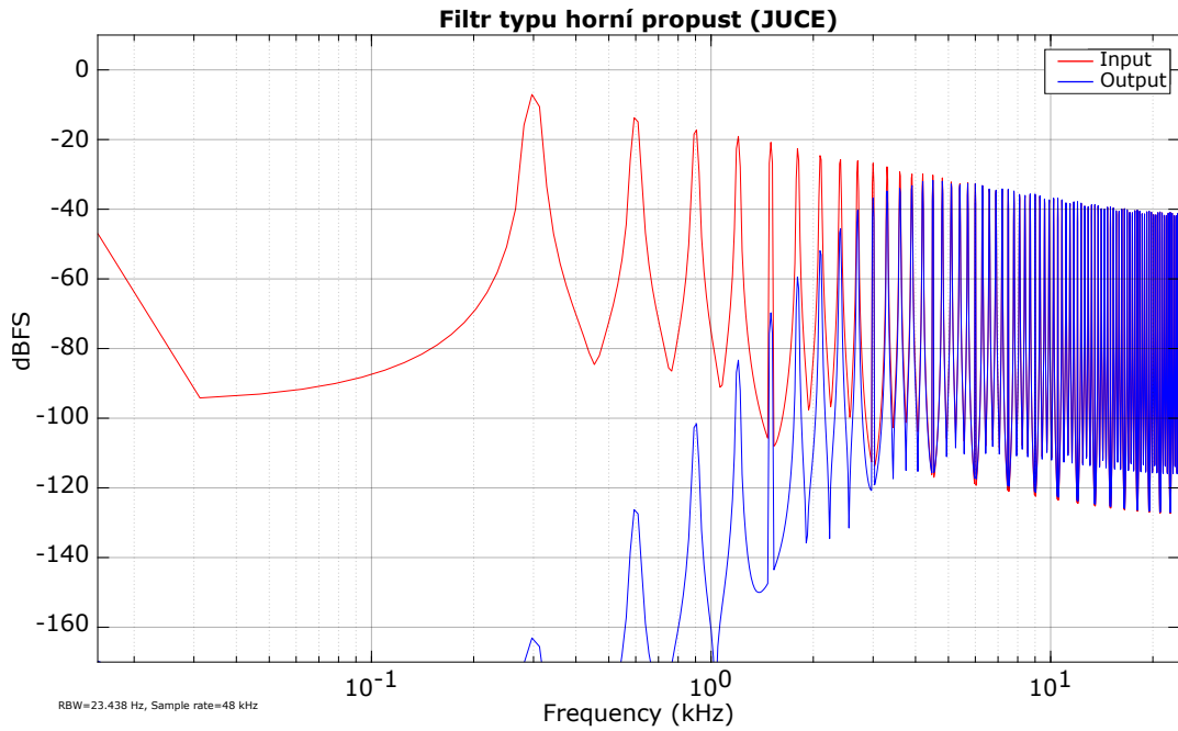
Obr. 3.22: Kmitočtové spektrum výstupního signálu po filtraci (horní propust).
