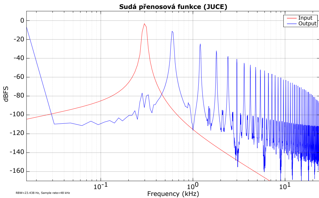
Obr. 3.18: Kmitočtové spektrum výstupního signálu po zkreslení (sudá funkce).
