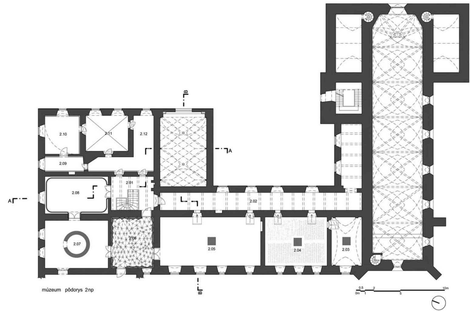
múzeum pôdorys 2:10
