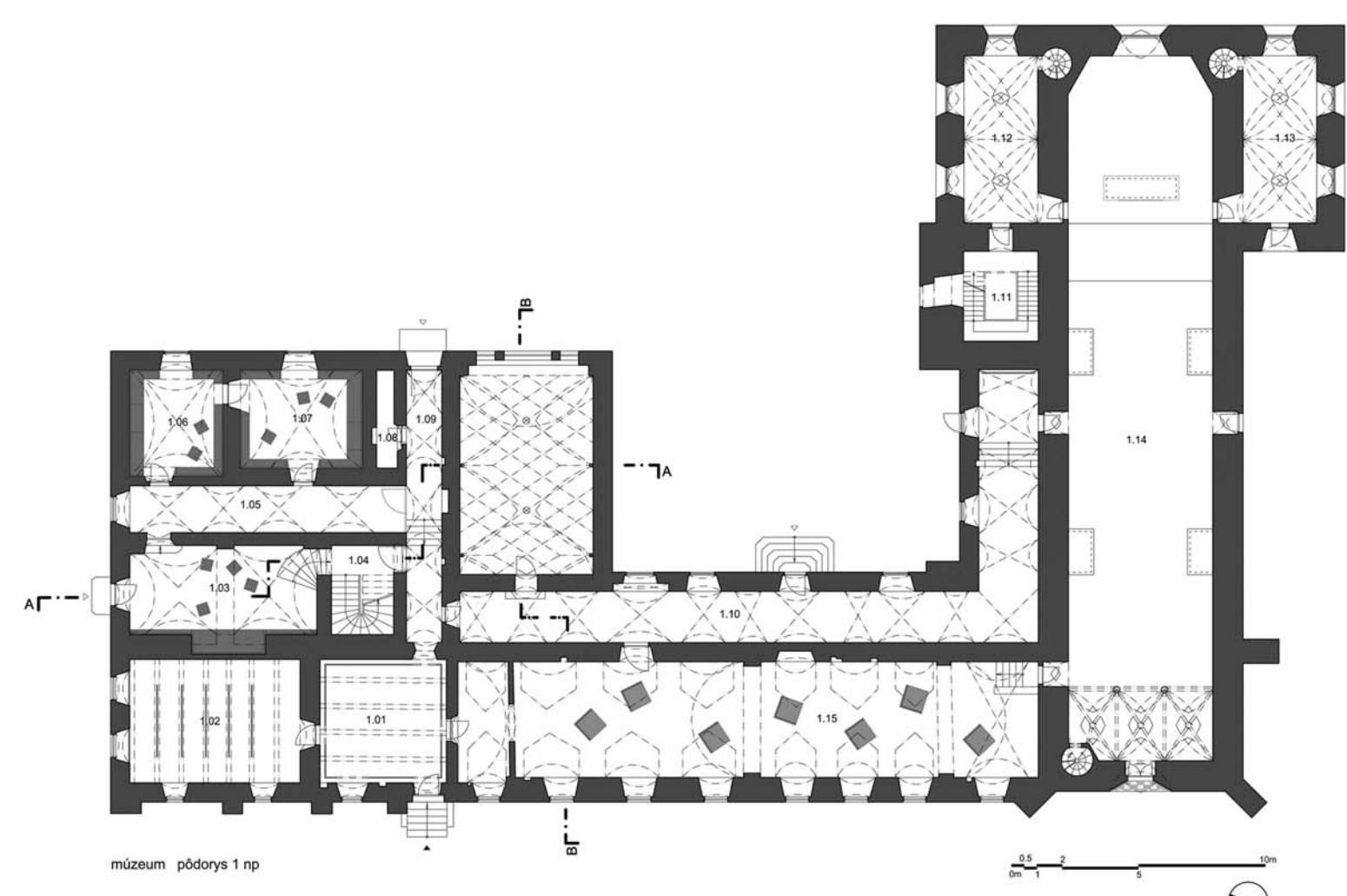
múzeum pôdorys 1:10
