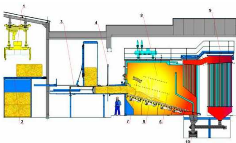
Obr. 4.8 Schéma kotle VESKO-S s popisem hlavní částí
