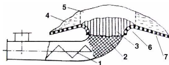
Obr. 4.4 Schéma spalovacího zařízení se spodním přívodem paliva
