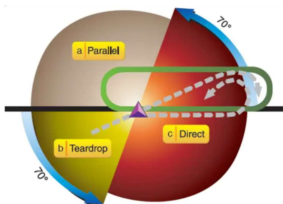
Obrázek 10 Vstupní sektory do vyčkávacího obrazce [21]
