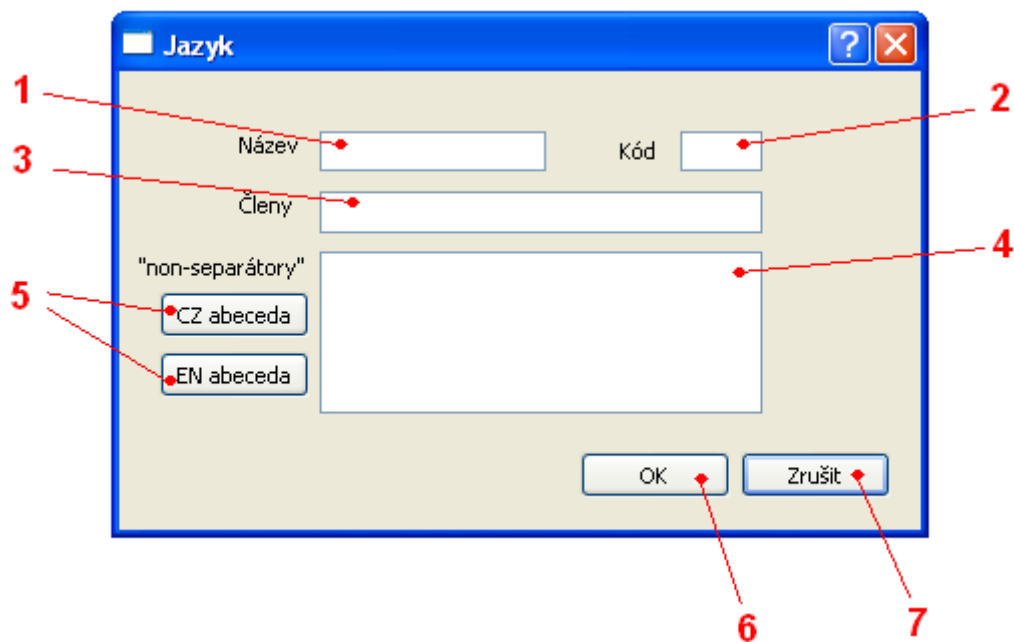
Obrázek 14 : Editor jazyka
