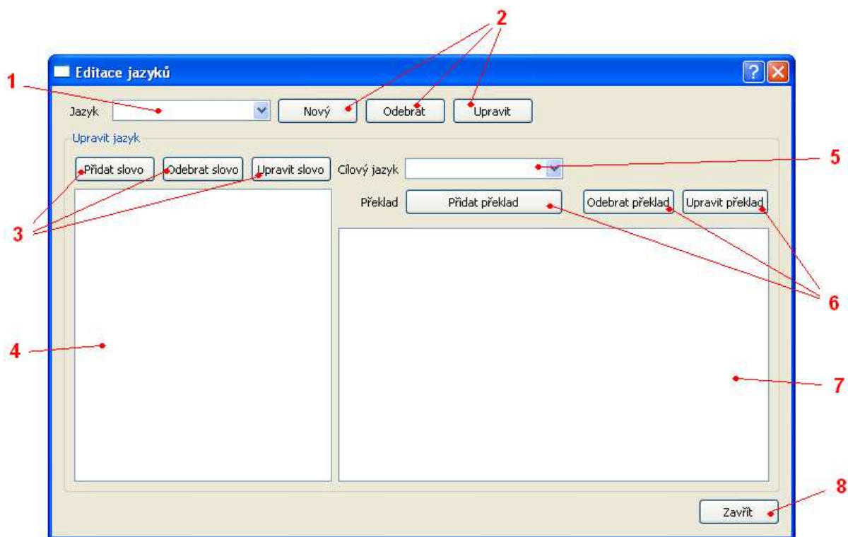
Obrázek 13 : Editace jazyků
