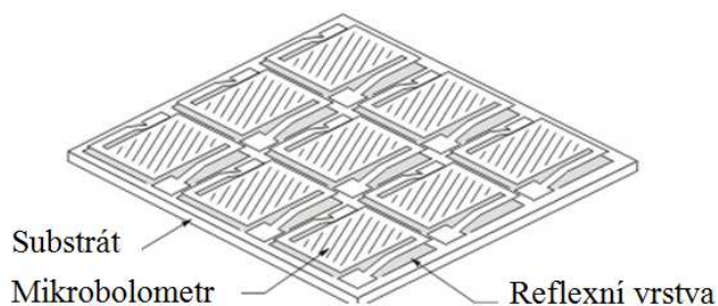
Obr. 11 Provedení mikrobolometru [13]
