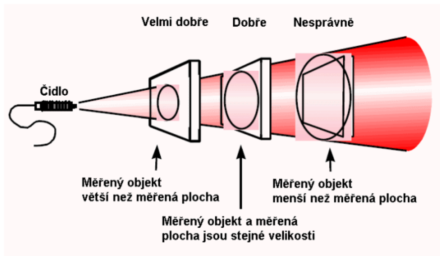
Obr. 13 Zaměření objektu [12]
