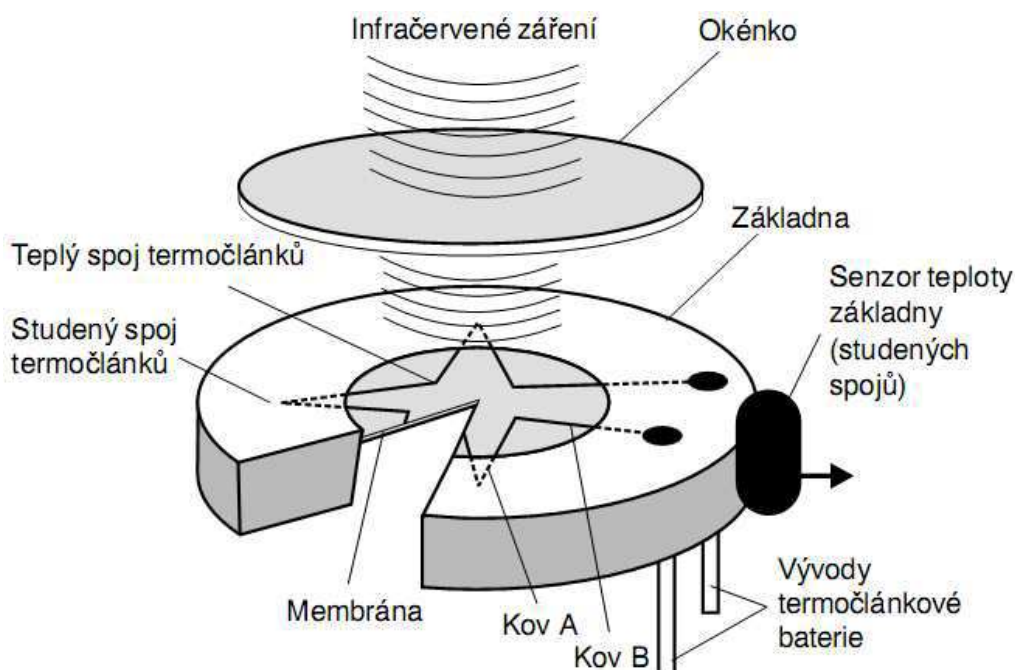
Obr. 9 Konstrukce tepelného detektoru s termočláneku [10]
