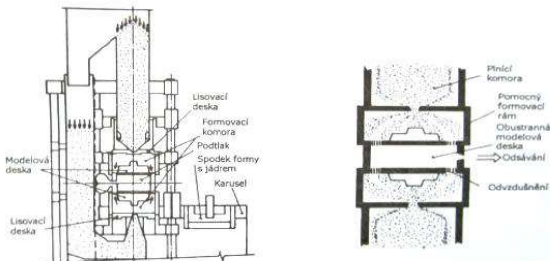
Obr. 8 Bezrámový formovací stroj DISA plnicí se podtlakem [7]
