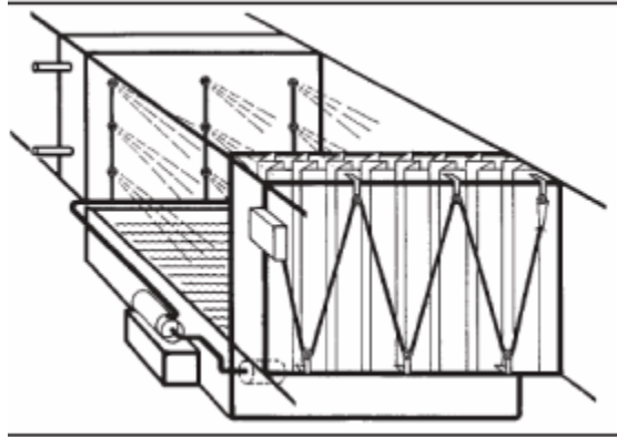
Obr. 14: pračka vzduchu [22]
