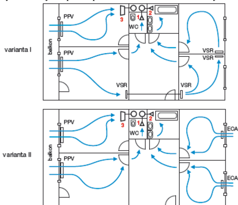
1 – elektricky ovládaný talířový ventil (24V nebo 230V); 2 – talířový ventil s mechanickým doběhem, který je možno umístit v Zóně 1 nad vanou; 3 – elektrický talířový ventil digestoře
