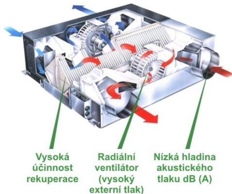
Obr. 10: integrovaná lokální rekuperační jednotka[18]
