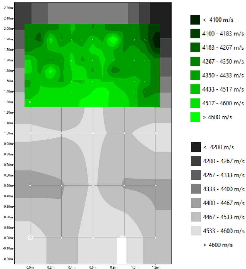
Obr. 2.42: Izovely podrobného měření sloupu II v kontextu základního rastru
