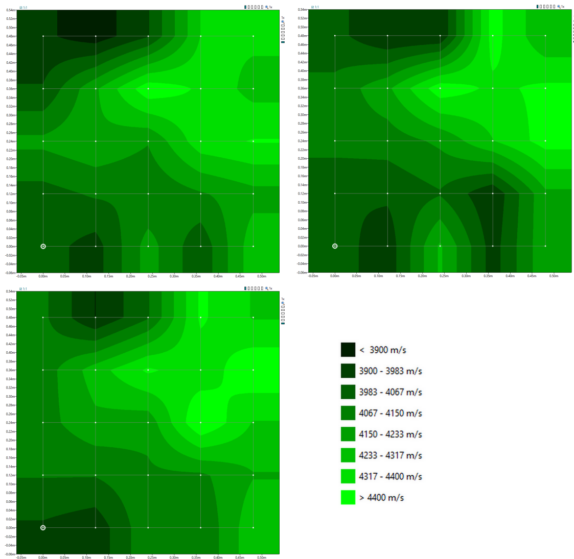
Obr. A.1: Izovely plošných skenů provedených sondami 82 kHz na zkušební desce
