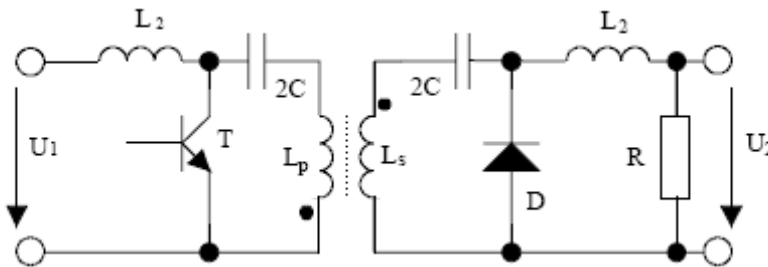
Obr. 7 - Zapojení Čukova měniče s oddělovacím transformátorem [1]
