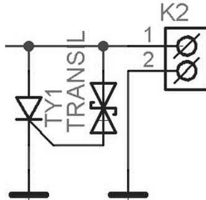
Obr. 27 – schéma zapojení přepětíové ochrany
