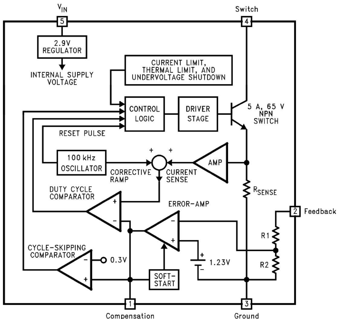
Obr. 25 – Blokový diagram obvodu LM2587 [5]
