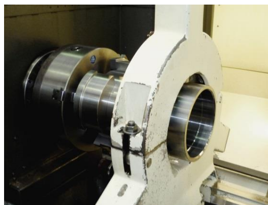
Obr. 3.9 Upnutý obrobek.
