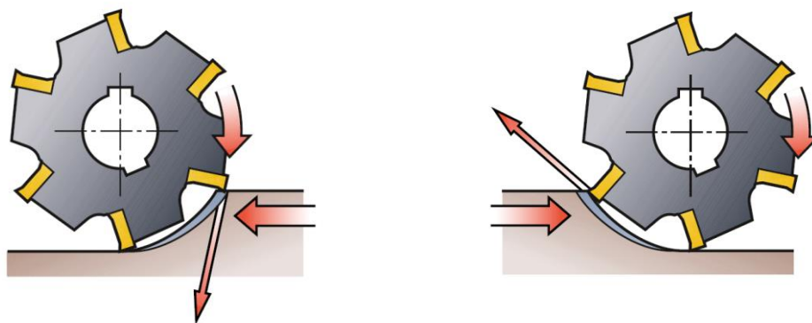
Obr. 2.5 Rozdíl mezi sousledným frézováním (vlevo) a nesousledným frézováním (vpravo) [8].
