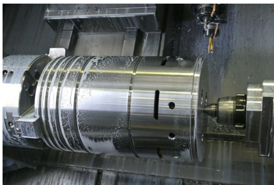
Obr. 3.15 Upnutý obrobek.
