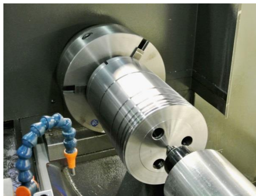
Obr. 3.11 Obrobek podepřený přes zátku.
