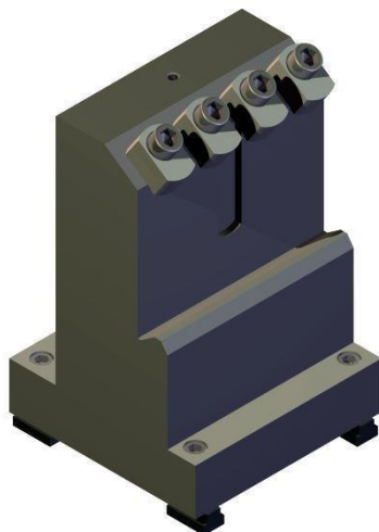
Obr. 4.3 Návrh sestavy upínacího přípravku.
