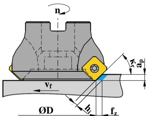
Obr. 2.10 Čelní frézování [14].
