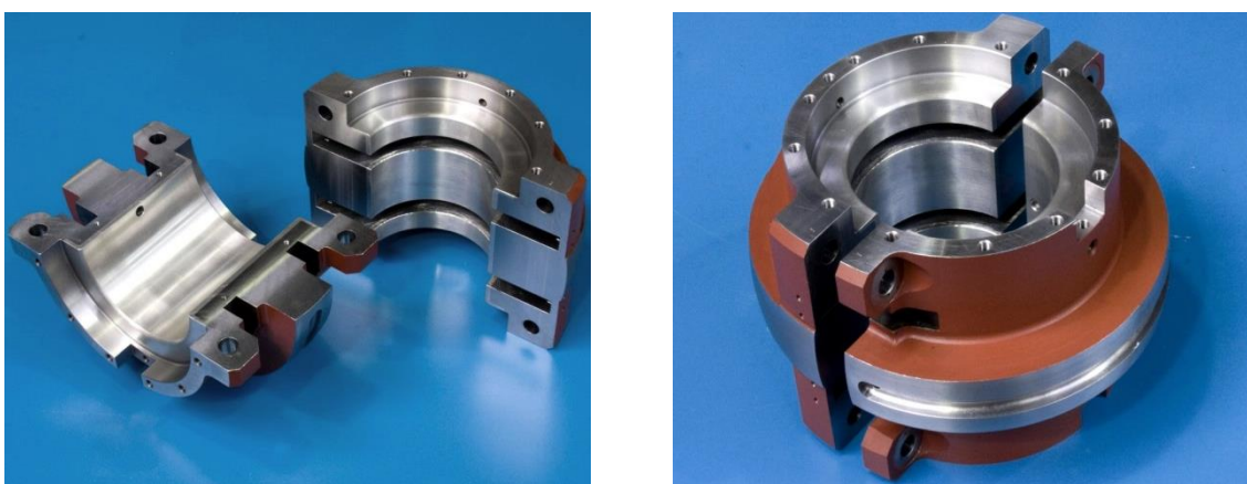
Obr. 1.4 Renovované ložisko [3].
