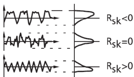
Obr. 2.4 Sklon profilu 16
