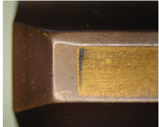
Obr. 4.11 Geometrie vodička nové vystružovací hlavice MT3
