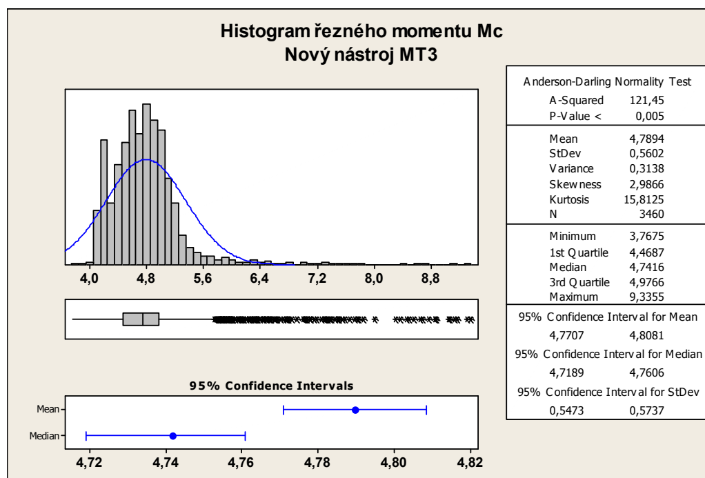
Obr. 4.16 Četnost řezného momentu M_c nového nástroje MT3
