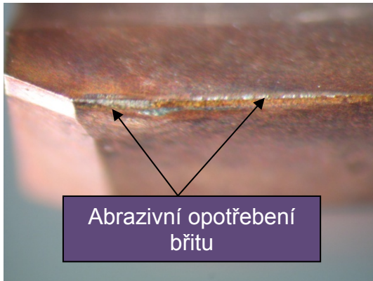
Obr. 4.12 Geometrie břitu opotřebované vystružovací hlavice MT3
