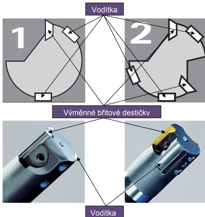
Obr. 1.2 Konstrukce nástrojů MAPAL 3
