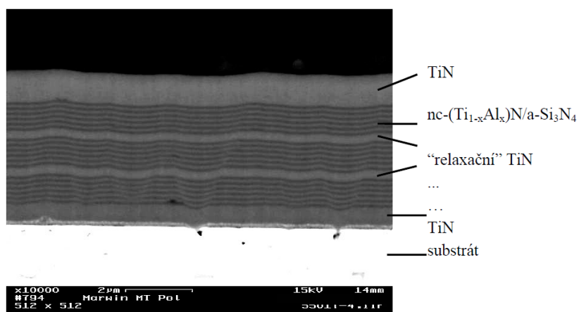
Obr. 1.4 Příklad nanokompozitního složení s multivrstvami firmy MARWIN 10
