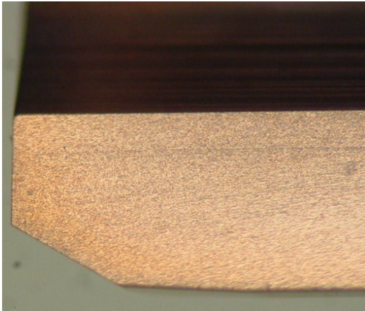
Obr. 4.10 Geometrie břitu nové vystružovací hlavice MT3
