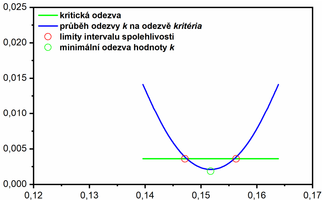
Obrázek 31 – Zobrazení průběhu odezvy rychlostní konstanty k na odezvě „Kritéria“ pro experiment uvolňování 6 mg·ml -1 sulfathiazolu
