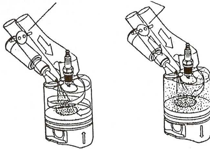
Obr. 5.3 – Řízení vzdušného proudění škrticí klapkou víření (Toyota D-4) [2]
