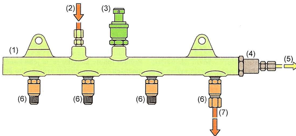
Obr. 4.3 – Zásobník paliva [1]
