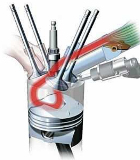
Obr. 1.1 – Vstřikovací systém Volkswagen FSI [5]
