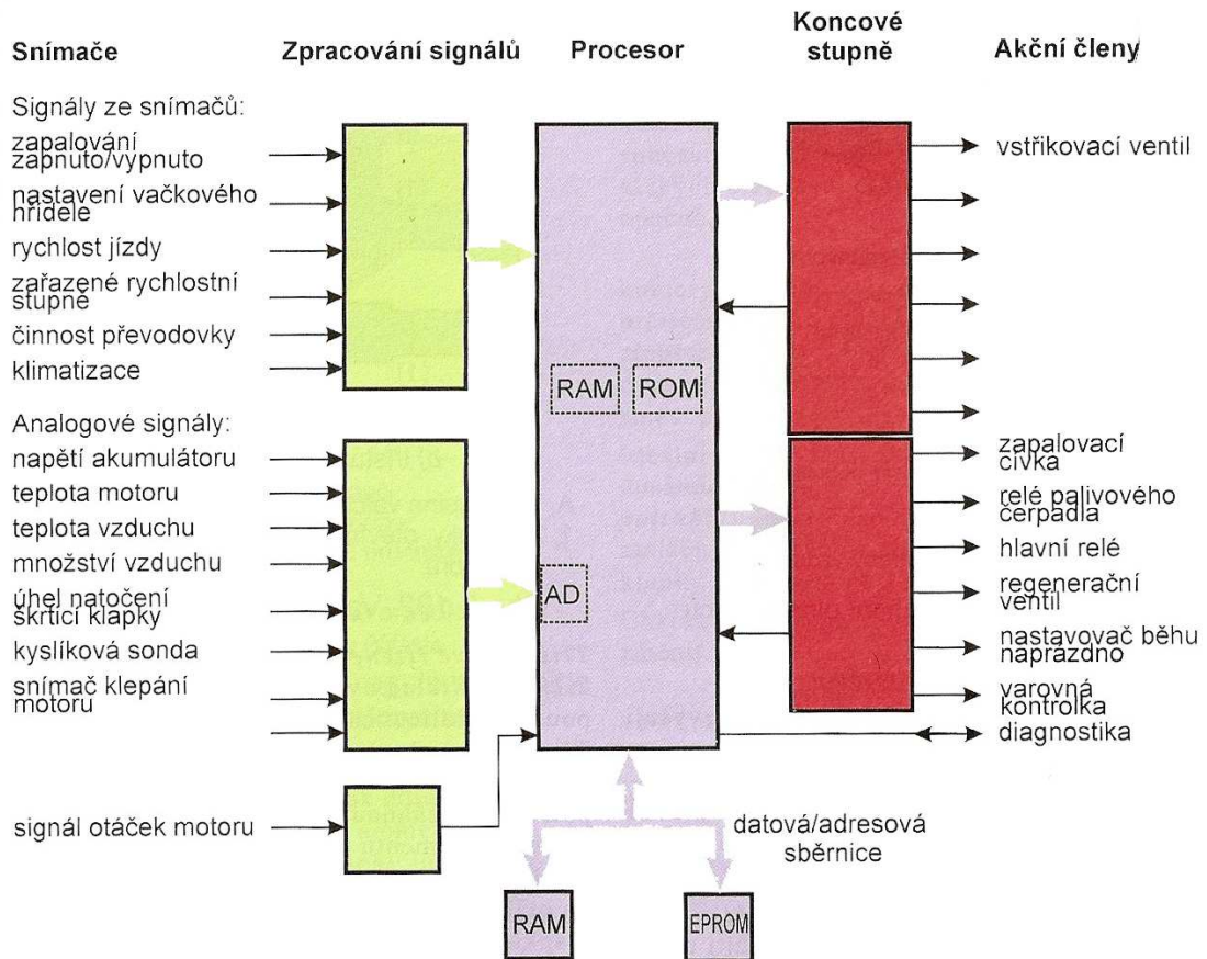
Obr. 4.6 – Blokové schéma řídicího systému [1]
