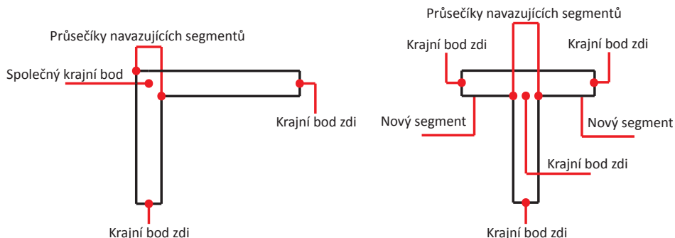
Obrázek 2.2: Napojování zdí
