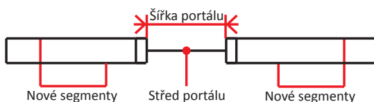
Obrázek 2.4: Vytváření portálů
