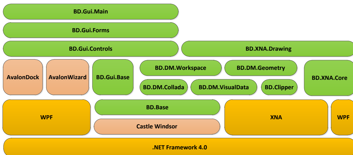
Obrázek 5.1: Architektura aplikace
