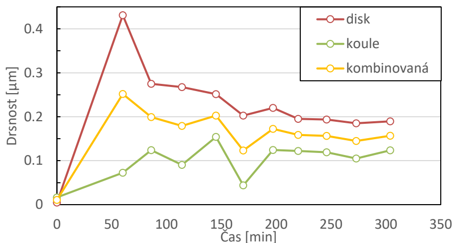
Obr. 5-16 Vývoj drsnosti v čase
