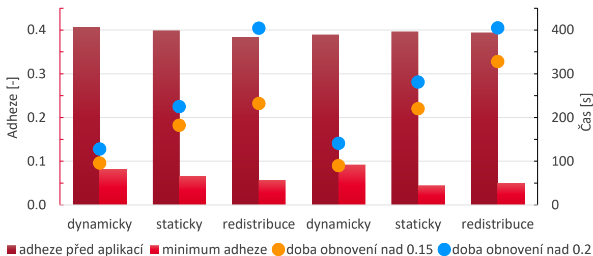
Obr. 5-6 Vliv způsobu aplikace pro 2 µl maziva
