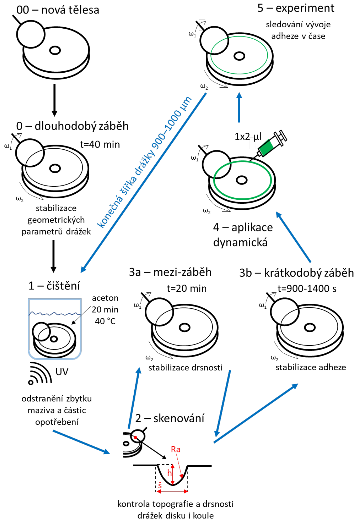
Obr. 5-29 Schéma navržené metodiky
