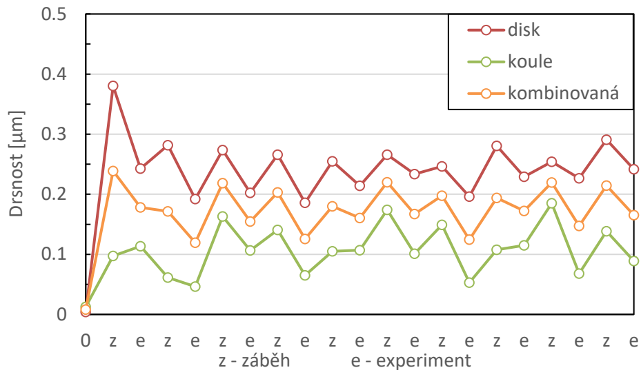
Obr. 5-18 Vývoj drsnosti pro 4 a 8 µl
