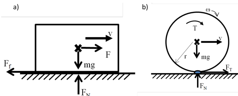
Obr. 2-2 Schéma a) čistého skluzu, b) valení - upraveno [5]
