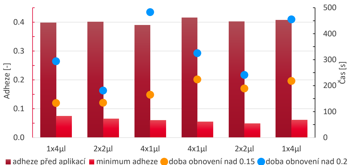
Obr. 5-9 Vliv dávkování do kontaktu pro 4 μl maziva
