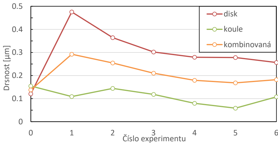
Obr. 5-26 Vývoj drsností při aplikaci oleje na zaběhlý disk
