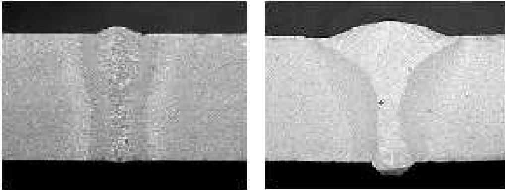
Obr. 5.2 Příčný výbrus I svaru zhotovený metodou svařování laserem (vlevo) a metodou Laser-Hybrid (vpravo)[5]
