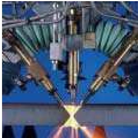
Obr. 6.4 Numericky nastavitelná hlava, uhel rozsahu 20°-49° [6]
