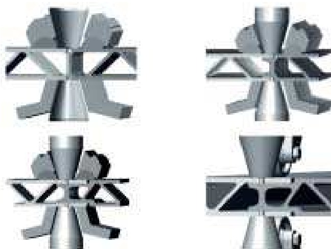
Obr. 6.1 Možnosti uspořádání svařovací hlavy [6]
