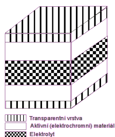
Obr. 2.1: Ukázka struktury elektrochromního zařízení
