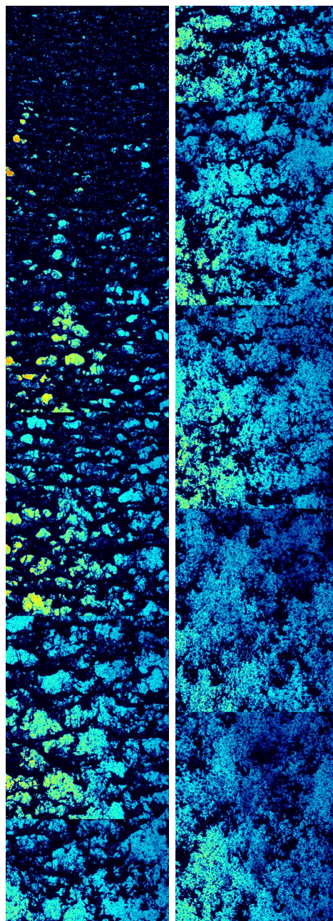
Obrázek 4.4: Složené stínografické fotografie vodního paprsku Trysky 8 od výšky 40 mm do 222 mm při tlaku 20 MPa; fotografie rozdělena na poloviny z důvodu velké délky
