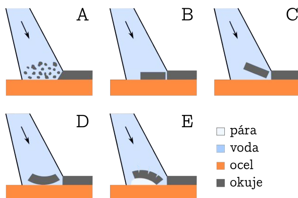
Obrázek 2.1: Fyzikální principy odstranění okují [10]
