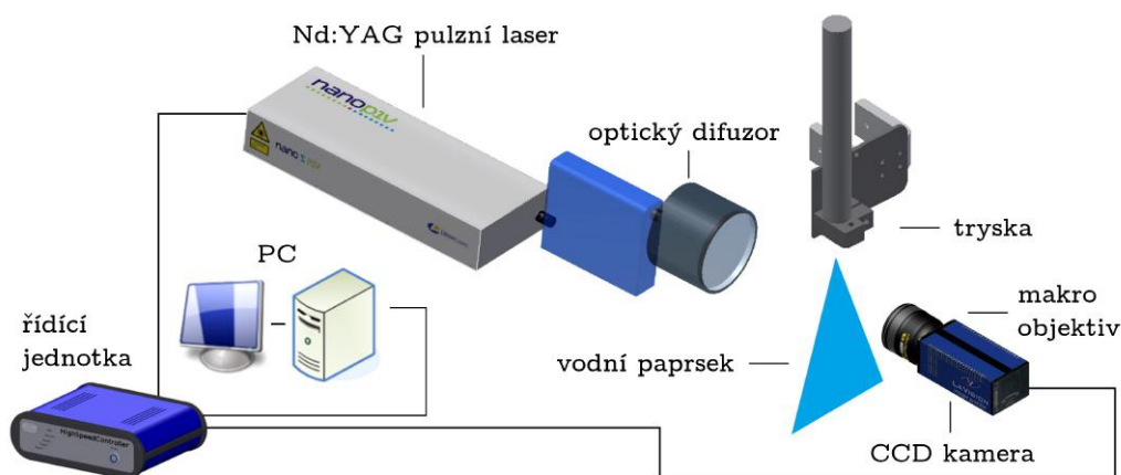
Obrázek 3.1: Princip pořizování fotografií stínografickou metodou [11]
