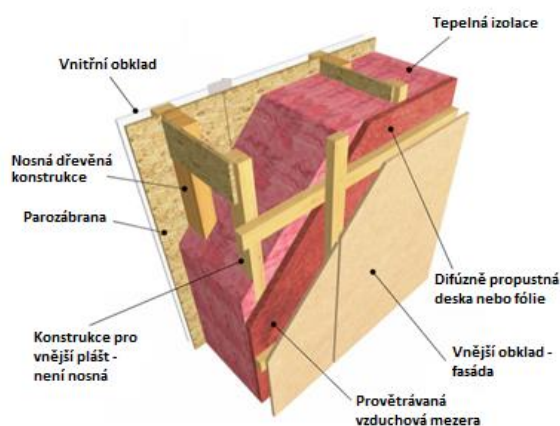
Obrázek 7: Skladba lehké provětrávané obvodové stěny [38]
