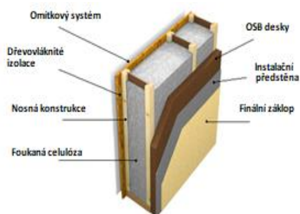
Obrázek 6: Skladba lehké neovětrávané obvodové stěny [37]
