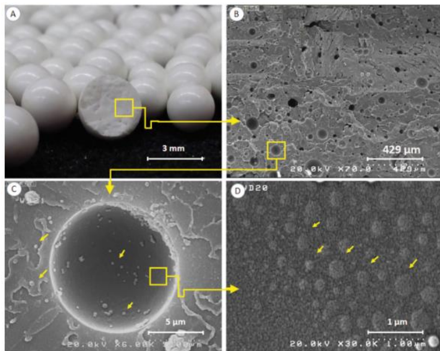
Obrázek 12: a) kompaktní kuličky CNFWEPS, b) průřez kompaktní kuličkou, c) místo kapiček vody, d) místo kapiček vody při větším zvětšení [50]
