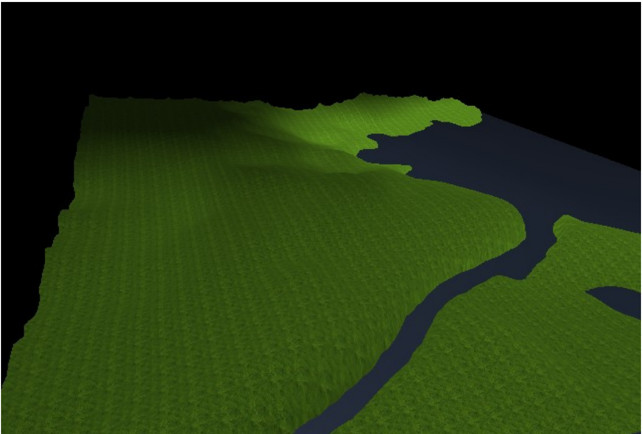
Obrázek 20: Řeka vlévající se do moře
