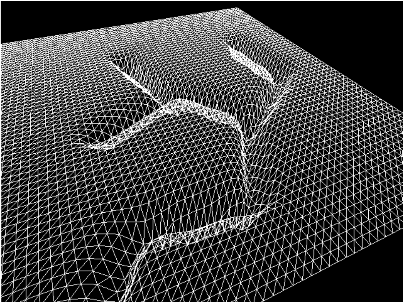
Obrázek 19: Síť řek vygenerovaná pomocí stochastického L-systému zapuštěná v rovině
