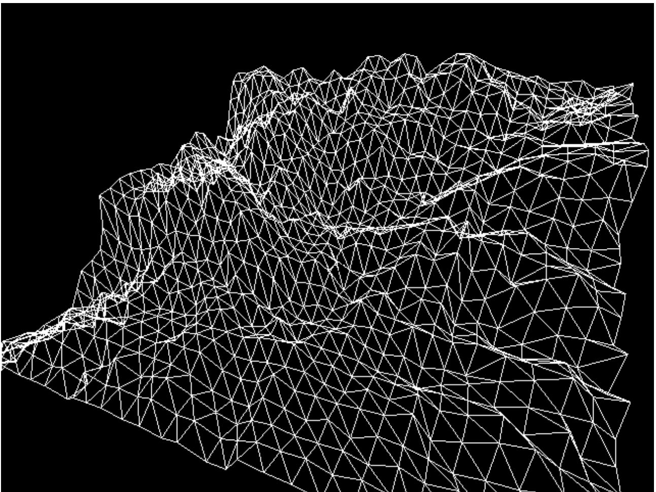
Obrázek 12: Algoritmus dělení roviny, 5000 iterací
