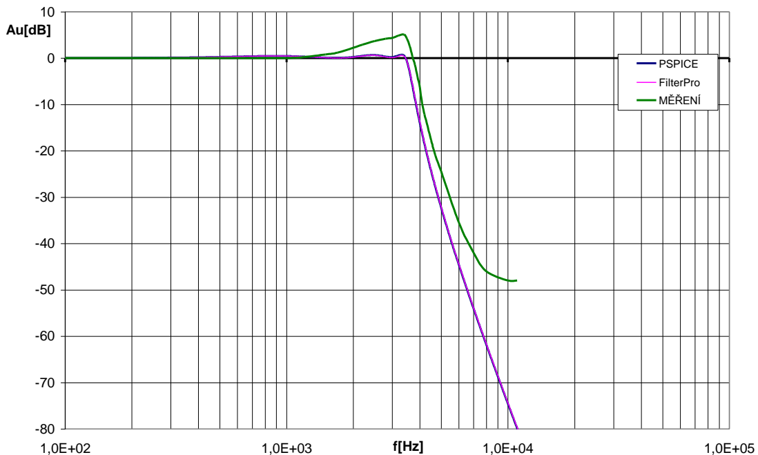
Obr. 3.2: Simulované a změřené frekvenční charakteristiky anti-aliasingového filtru.
