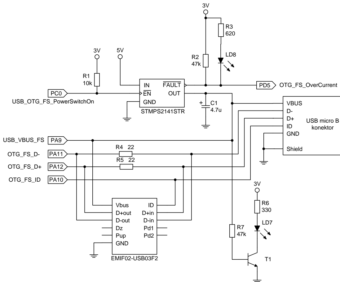
Obr. 4.1: Připojení USB konektoru k MCU (převzato z [11]).
