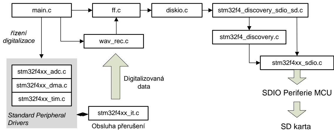
Obr. 6.1: Struktura souborů pro zápis na SD kartu.
