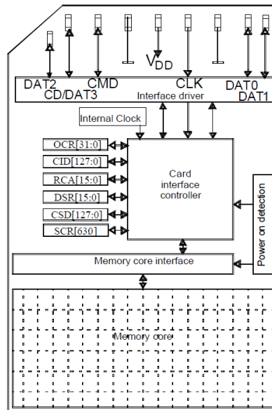
Obr. 5.2: Architektura SD karty. (převzato z [13])
