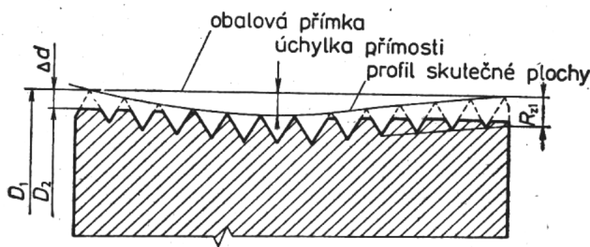
Obr. 1.3 Schéma kalibrace plochy s úchytkami přímosti [8]
