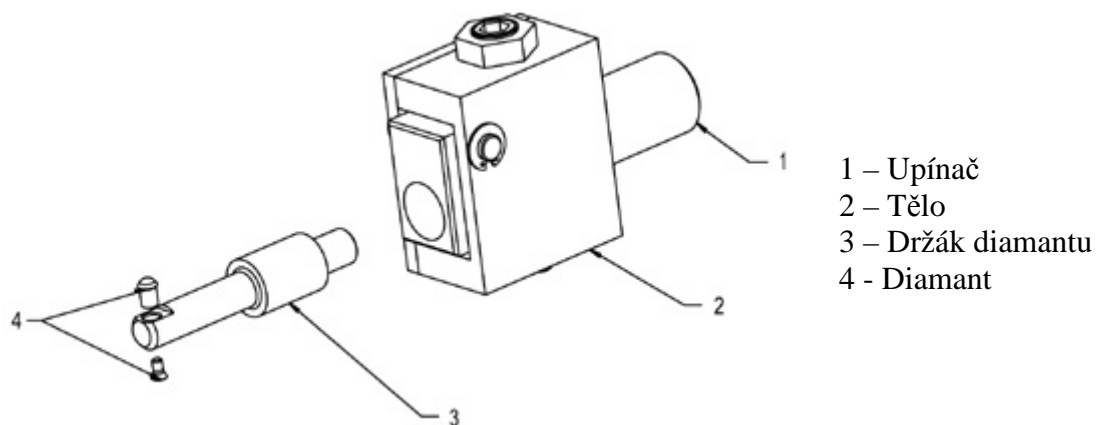
Obr. 2.20 Náhradní díly diamantového hladicího nástroje [13]
