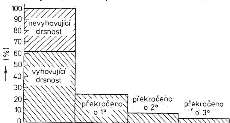
Obr. 4.3 Podíl nevyhovujících drsností (%) z celkového počtu kontrolovaných ploch [8]
