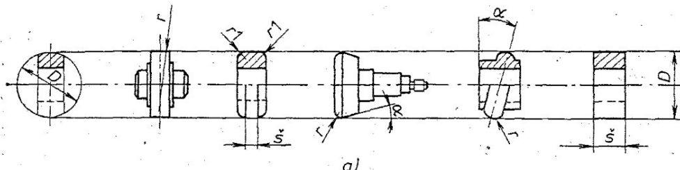
Obr. 1.5 Geometrické tvary tvářecích prvků [8]
