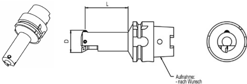
Obr. 2.24 Více funkční nástroj pro třískové obrábění a hlazení v jedné výrobní operaci [10, 13]
