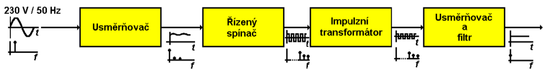
Obrázek 2.2: Blokové schéma spínaného zdroje [1]
