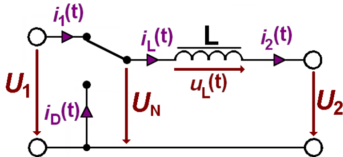
Obrázek 3.7: Pracovní cyklus 1 - sepnutý tranzistor T [4]
