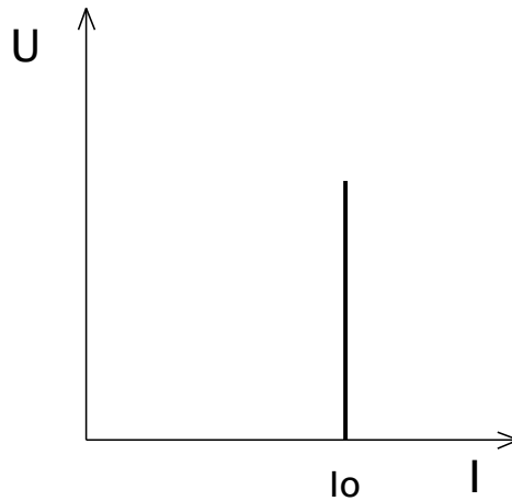
Obrázek 2.4: Zatěžovací charakteristika proudového zdroje
