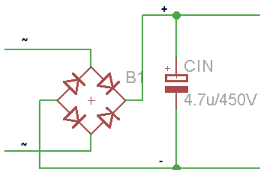
Obrázek 4.3: Schéma usměrňovače
