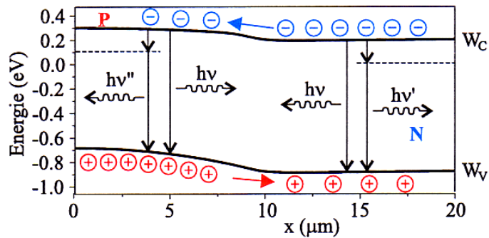
Obrázek 1.3: Princip elektroluminiscence [11]
