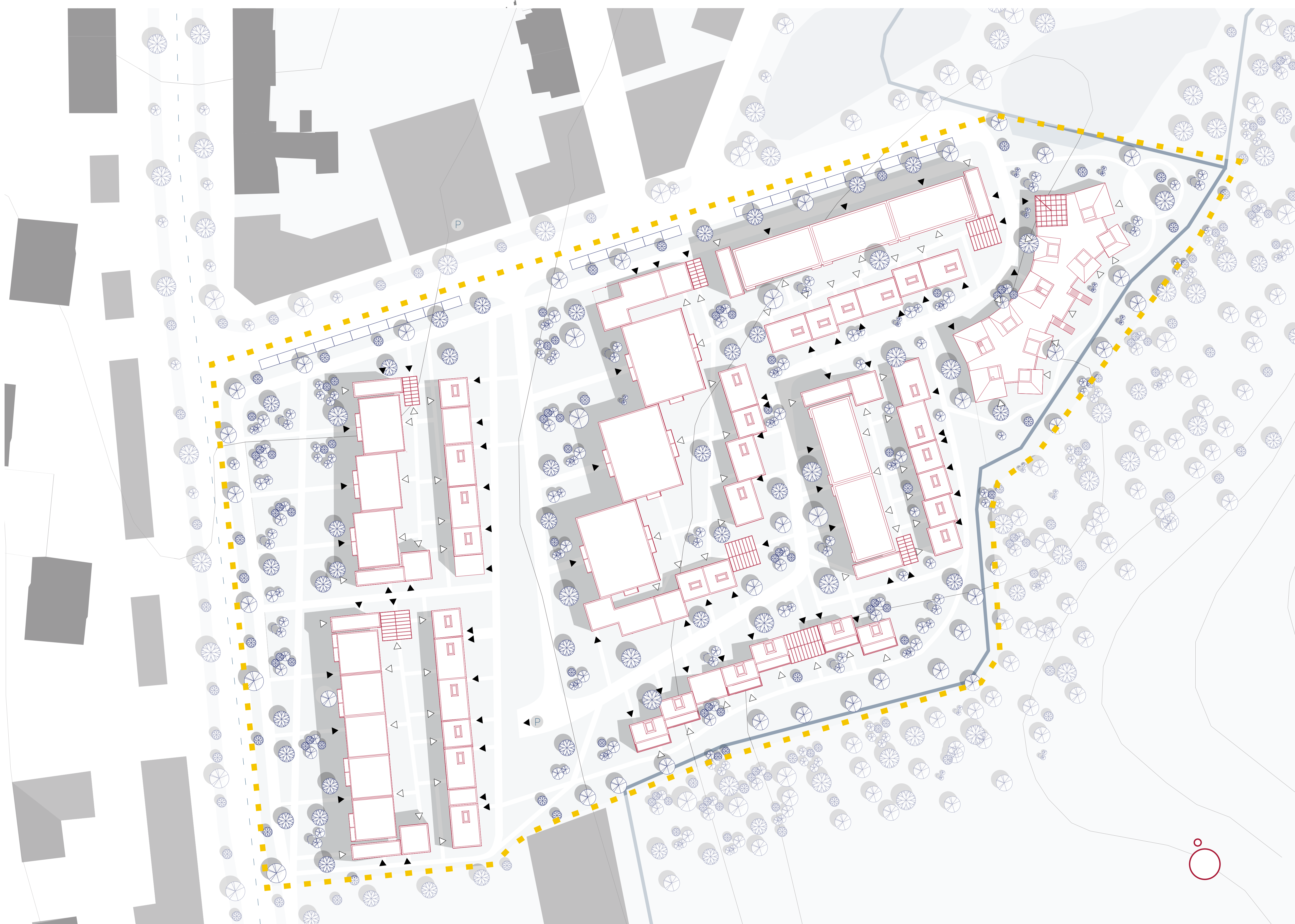
SITUACE 1:500
