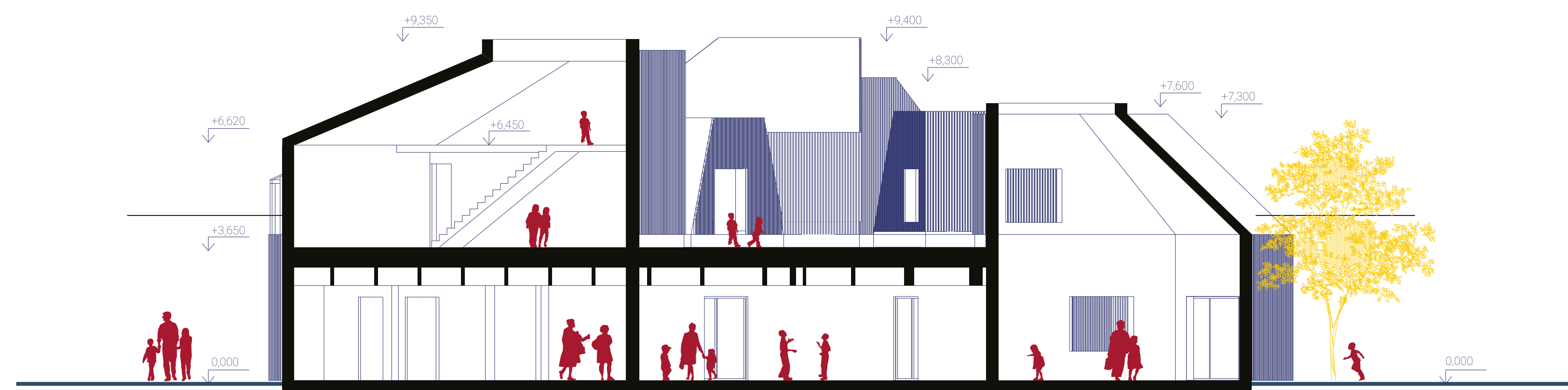
ŘEZ B-B 1:100
