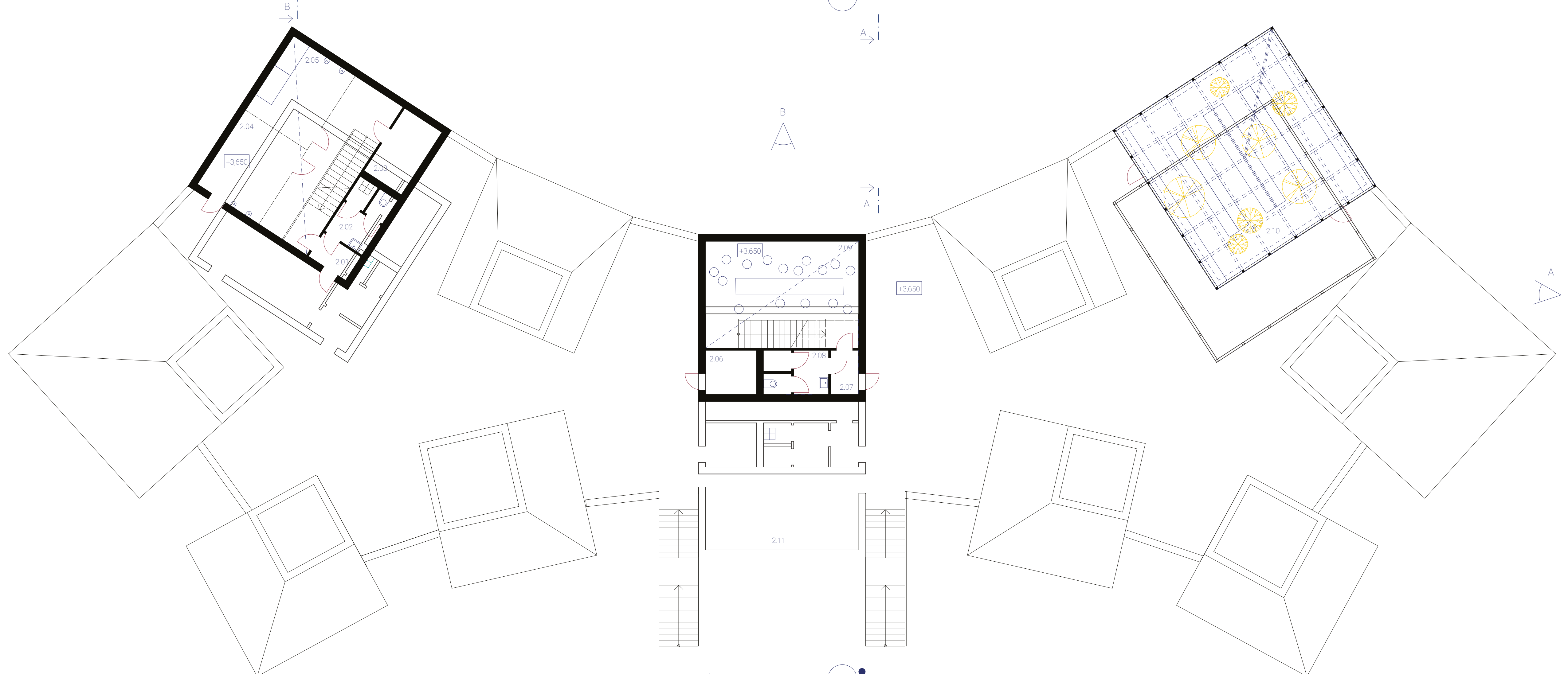
PŮDORYS 2NP 1:100
