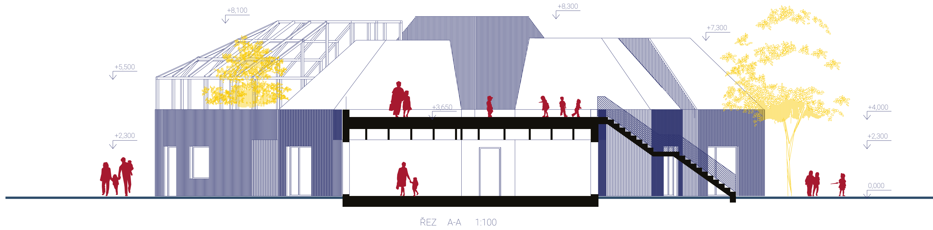
ŘEZ A-A 1:100
