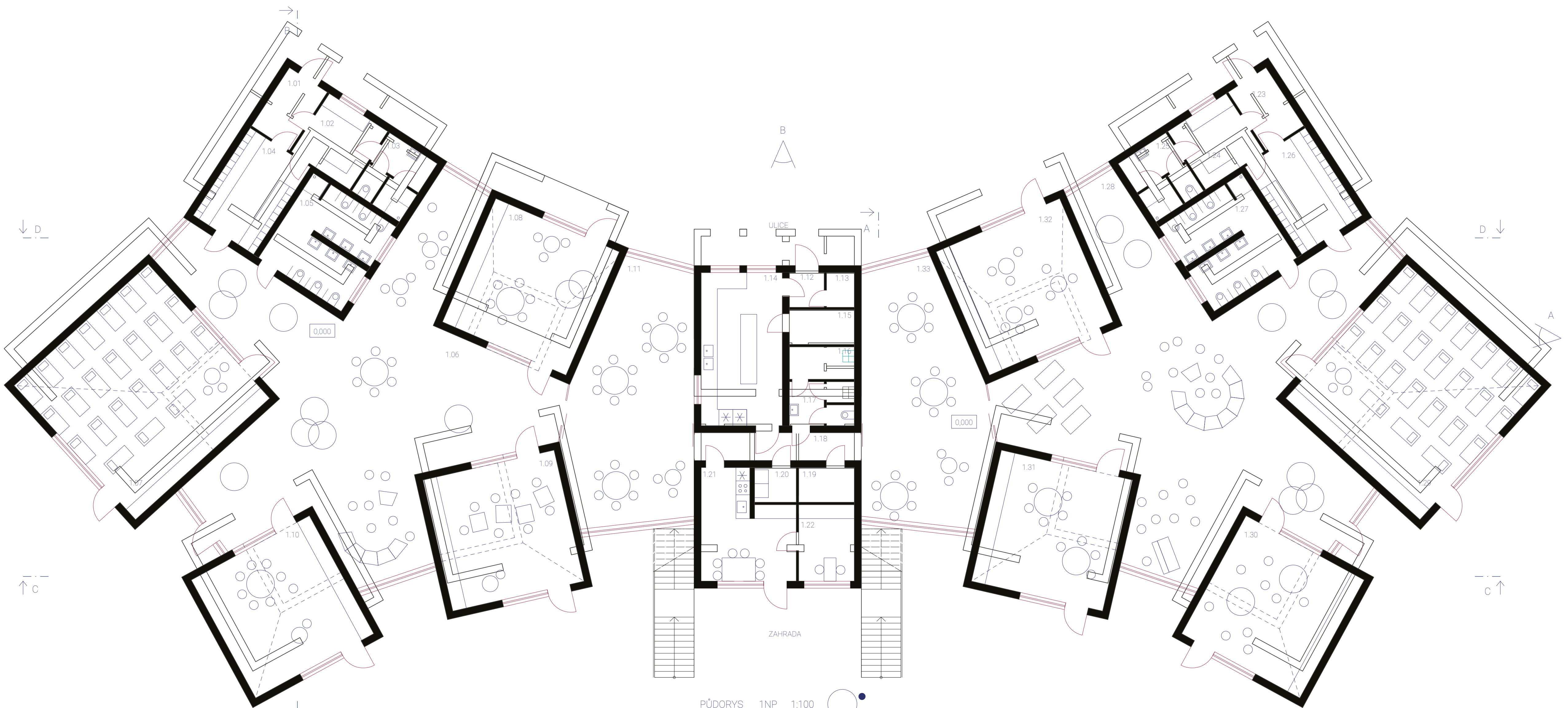
PŮDORYS 1NP 1:100
