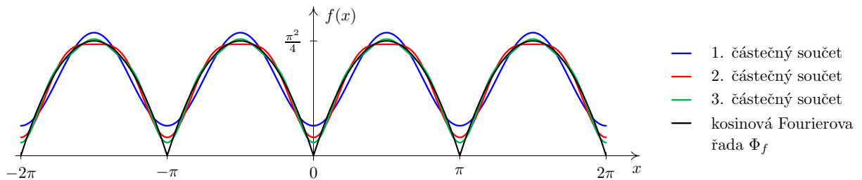
Obrázek 5.5: Graf vybraných částečných součtů a kosinové Fourierovy řady \Phi_f funkce f(x) = x(\pi - x)
