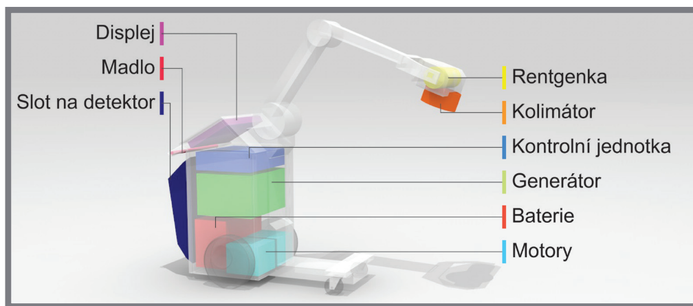
Obr. 2-1 schéma rentgenu
