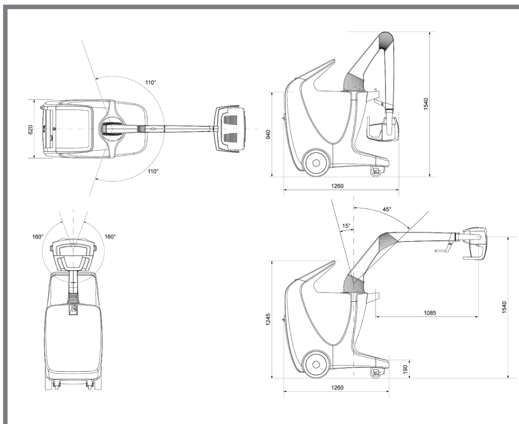
Obr. 8-1 Základní rozměry
