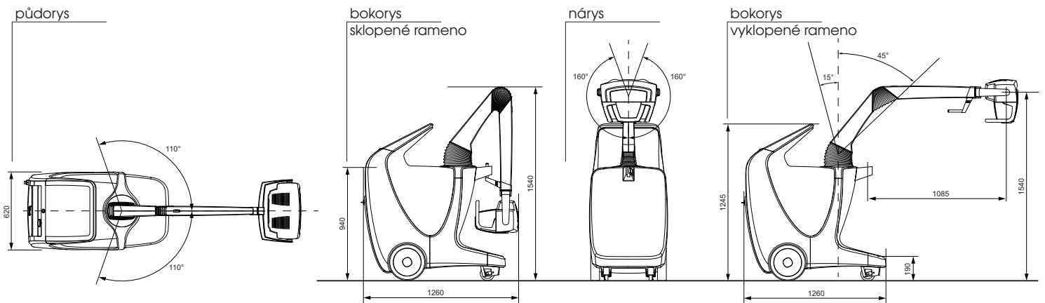
Technický náčrt - (M 1:15, mm)
