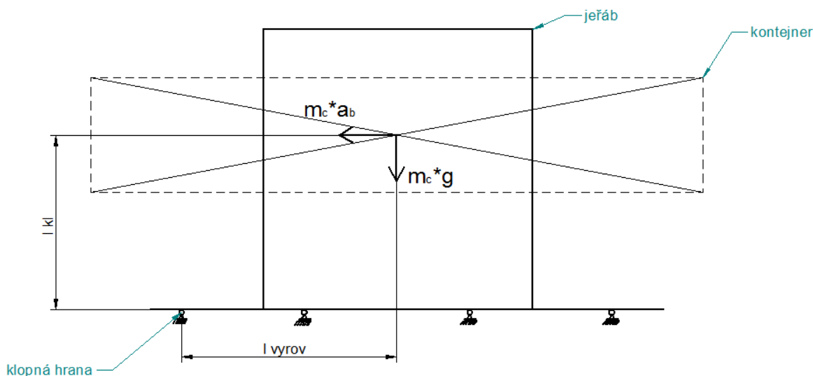
Obr. 7 Znárodnění klopících a vyrovnávacích sil
