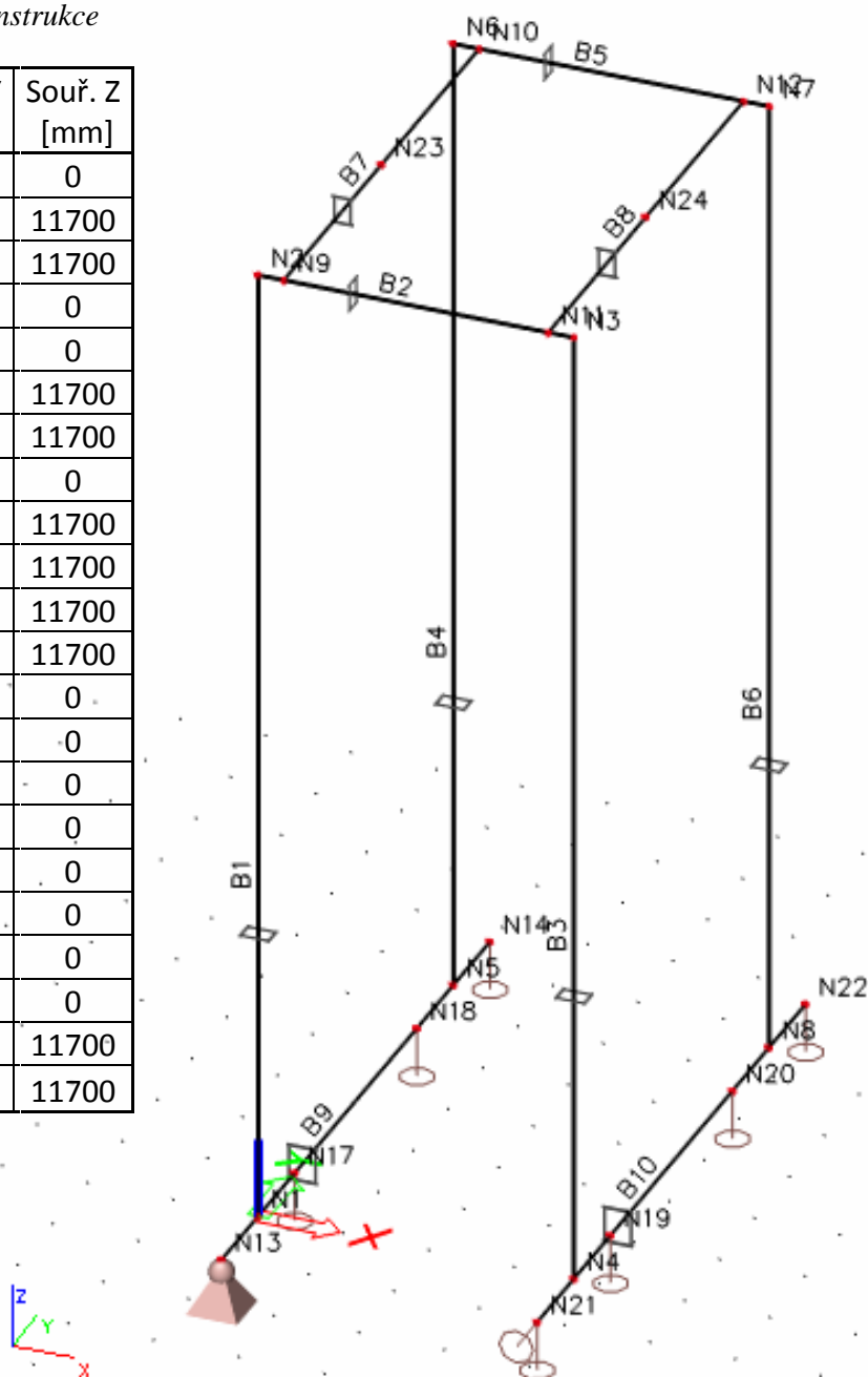
Obr. 9 Model konstrukce v programu SCIA ENGINEER
