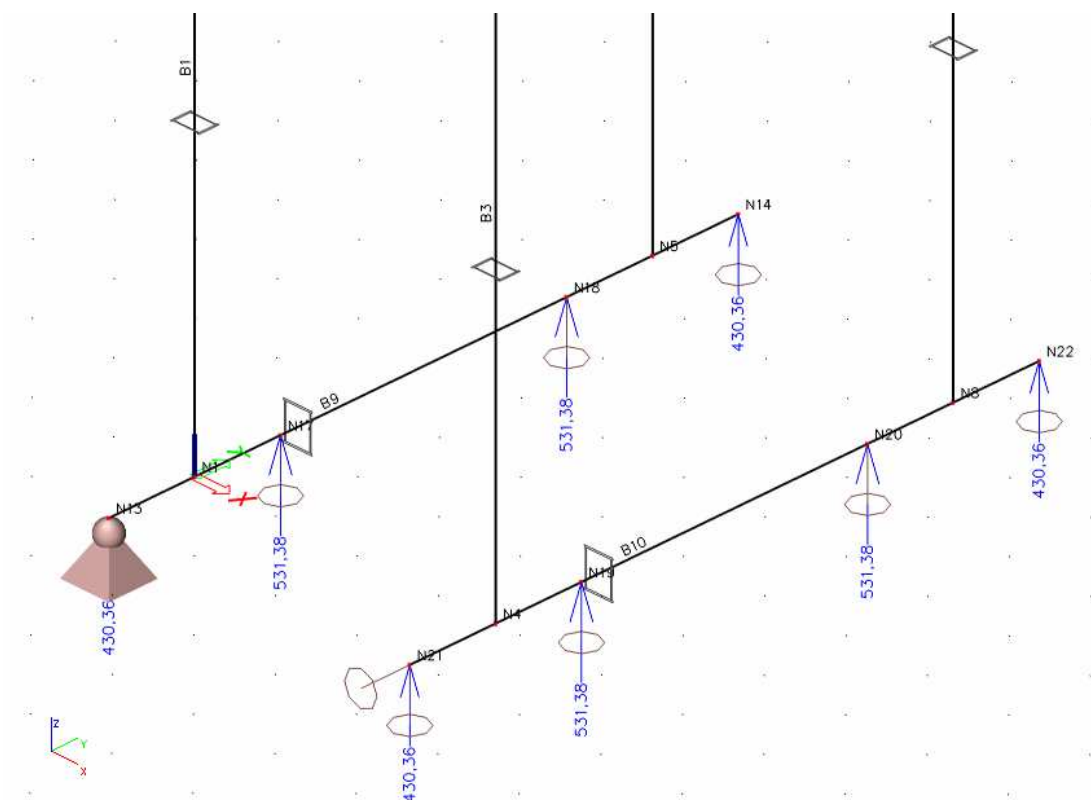
Obr. 11 Reakce v podporách
