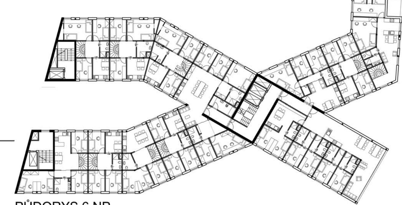
PŮDORYS 6.NP
