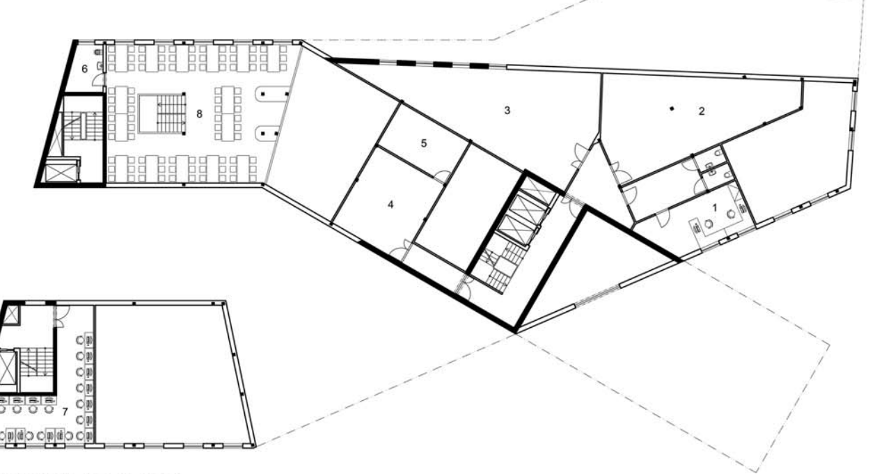
PŮDORYS 2.NP
