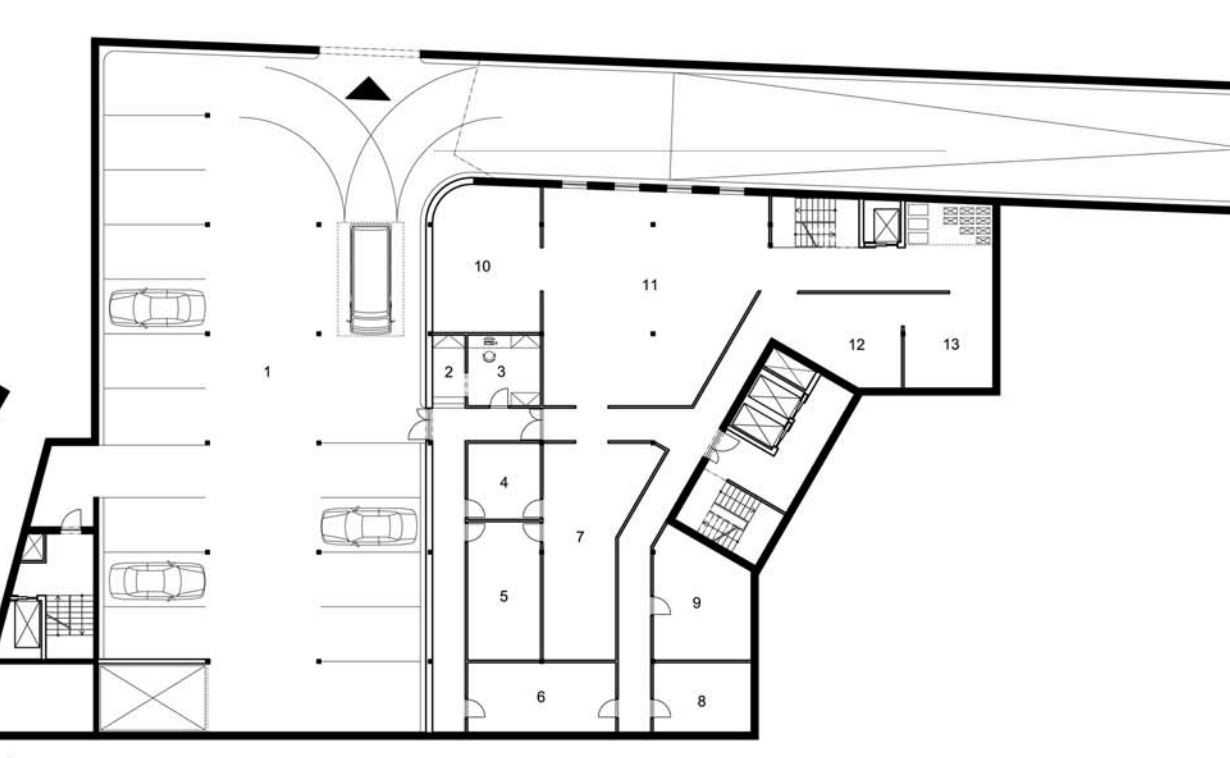
PŮDORYS 1.PP
