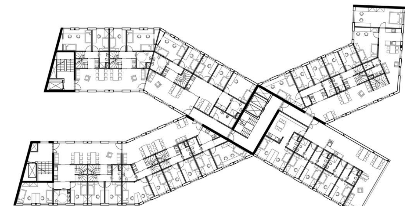
PŮDORYS 5.NP
