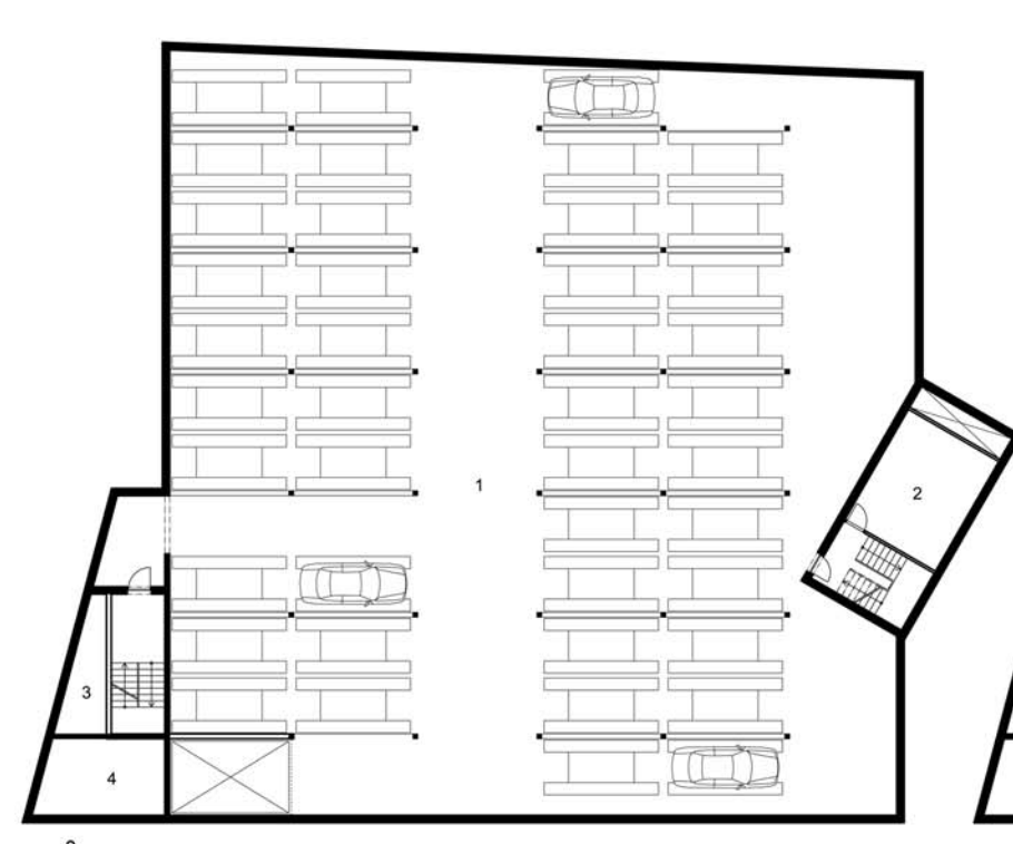
PŮDORYS 3.PP
