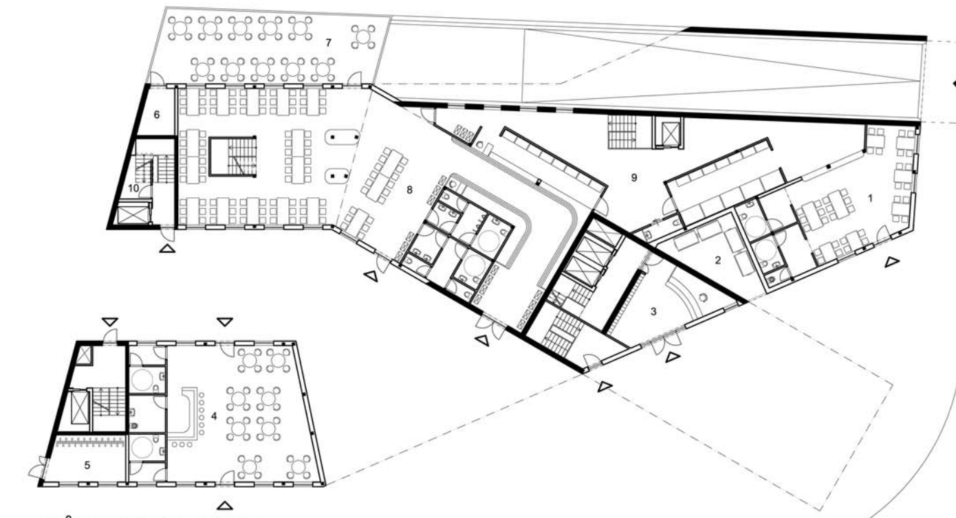
PŮDORYS 1.NP
