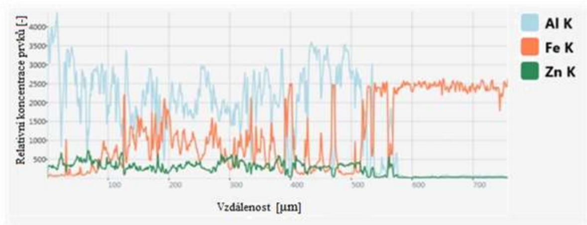
Obr. 7.17 Graf EDX Linescan přesného vysekávání
