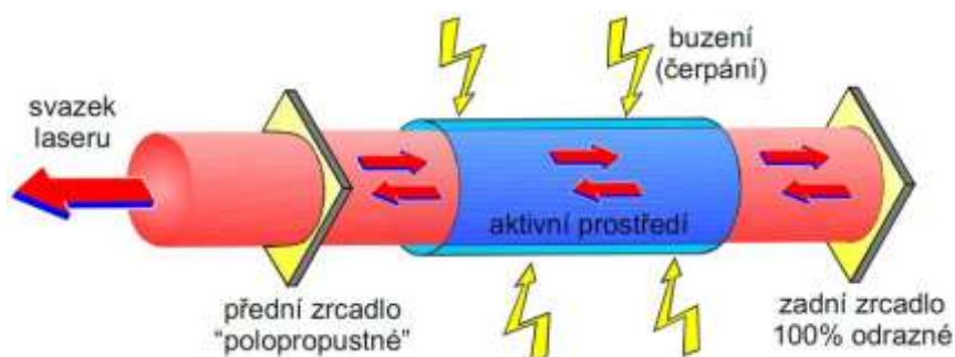
Obr. 2.1 Schematicky znázorněný optický rezonátor [24]
