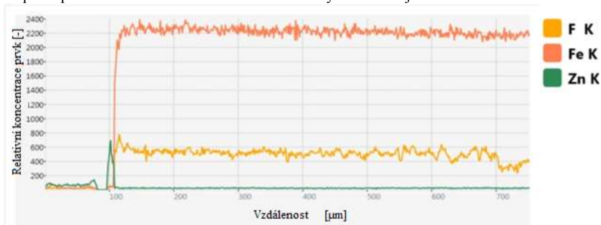
Obr. 7.9 Graf EDX Linescan laserového řezu
