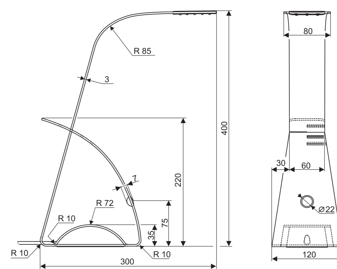
definující pohledy - měřítko 1:4, údaje v mm
