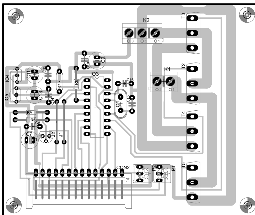
Obr. A.3: Deska plošných spojů DPS02 - pohled ze strany součástek.
