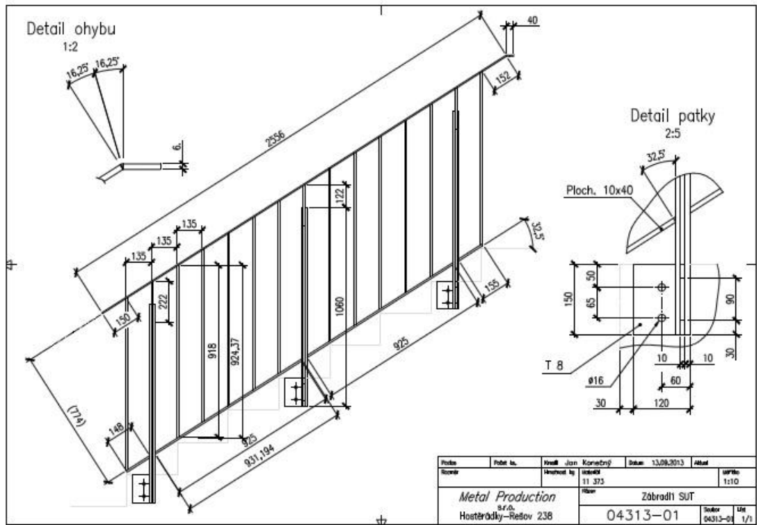
Obrázek 8 – Zábradlí schodiště
