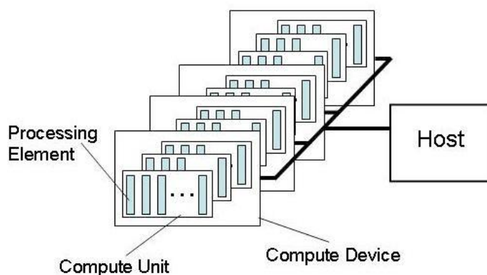
Obrázek 17: Model platformy: Jeden host, s jedním nebo více výpočetními zařízeními. Každé s jednou nebo více výpočetními jednotkami, každá s jedním nebo více procesními elementy
