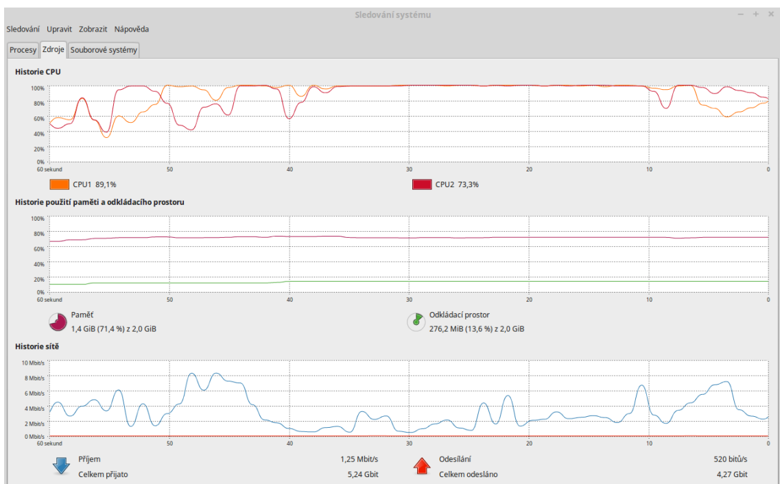
Obr. 3.11: Přetížení systému po spuštění mixu/translátoru vysoký bitový tok
