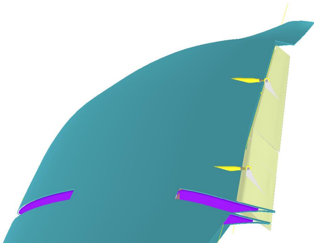
Obr. 11 Pohled na křídlo – klapky dolů + křídélka doleva
