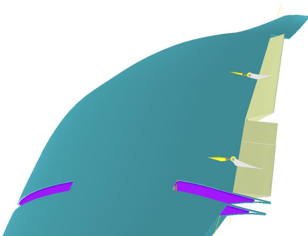
Obr. 10 Pohled na křídlo – klapky nahoru + křídélka doprava
