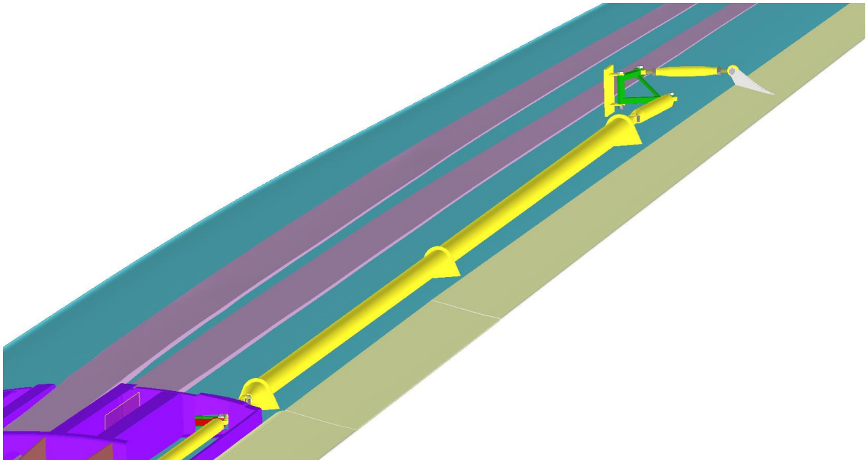
Obr. 3 Pohled na mechanismus náhonu vnějšího flaperonu ve vnějším segmentu křídla
