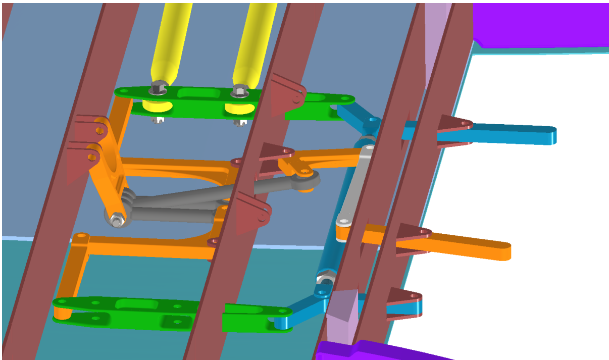
Obr. 1 Pohled na mixážní mechanismus a táhla náhonů flaperonů
