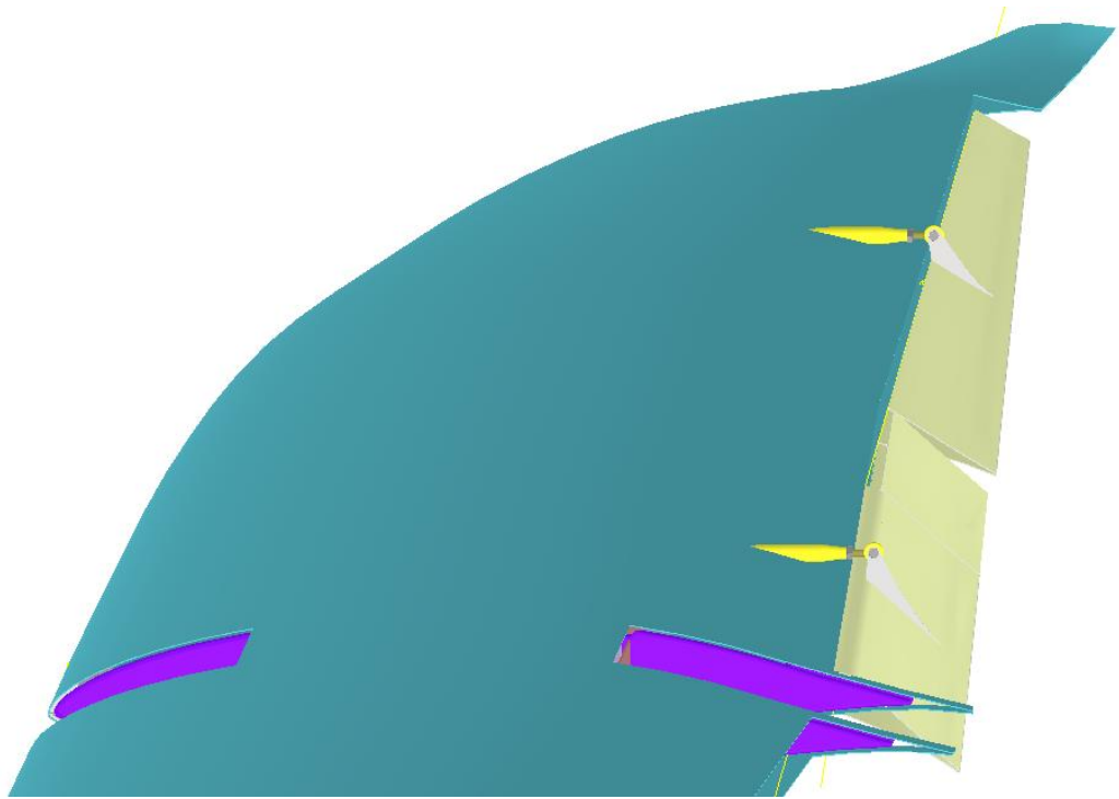
Obr. 7 Pohled na křídlo – klapky dolů
