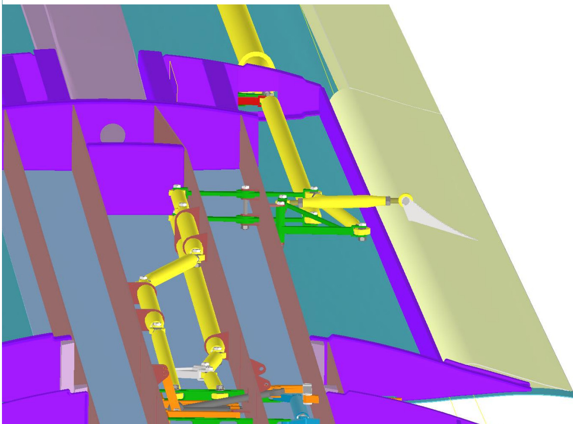
Obr. 2 Pohled na mechanismy náhonů flaperonů ve vnitřním segmentu křídla
