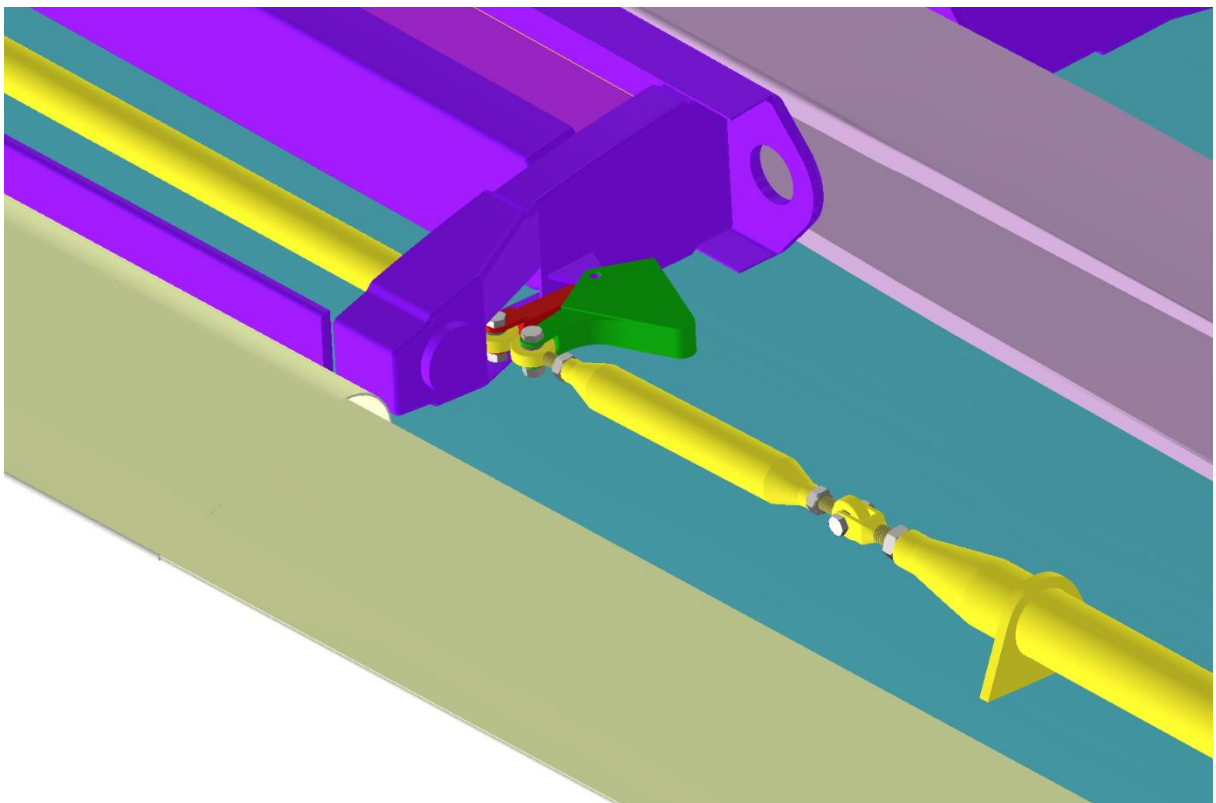
Obr. 4 Pohled na mechanismus automatického propojení soustav řízení mezi vnitřním a vnějším segmentem křídla
