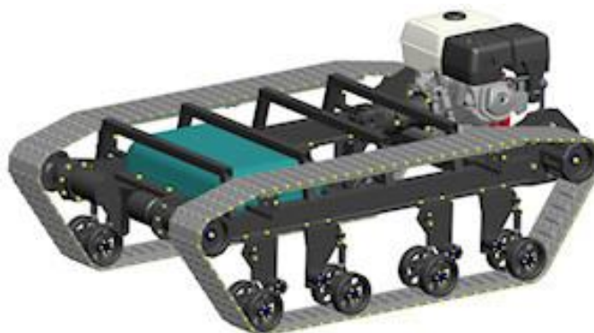
Obr. 24 Pásový podvozek (42)
