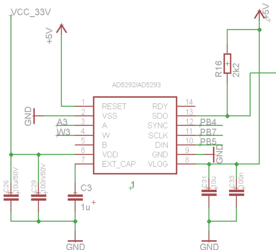
Obr. 16: Zapojení digitálního potenciometru
