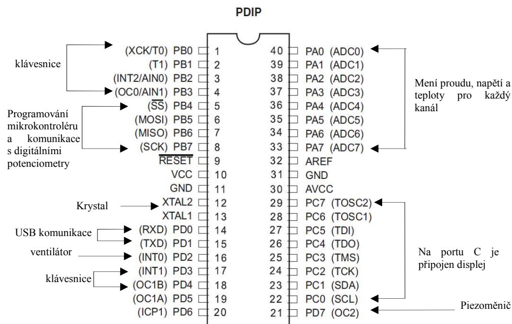
Obr. 4 : Využití vývodů mikrokontroléru (převzato z [4])
