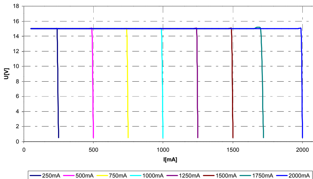
Obr. 29 : Měření proudové pojistky
