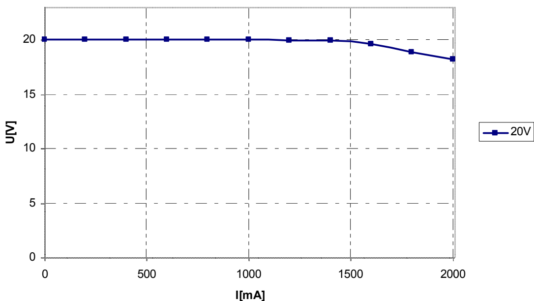
Obr. 28 : Zatěžovací charakteristika zdroje
