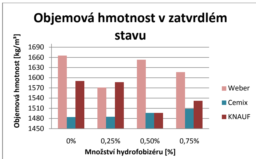
Graf 10 Objemové hmotnosti v zatvrdlém stavu [ \text{kg}/\text{m}^3 ] u zkoušených druhů omítek
