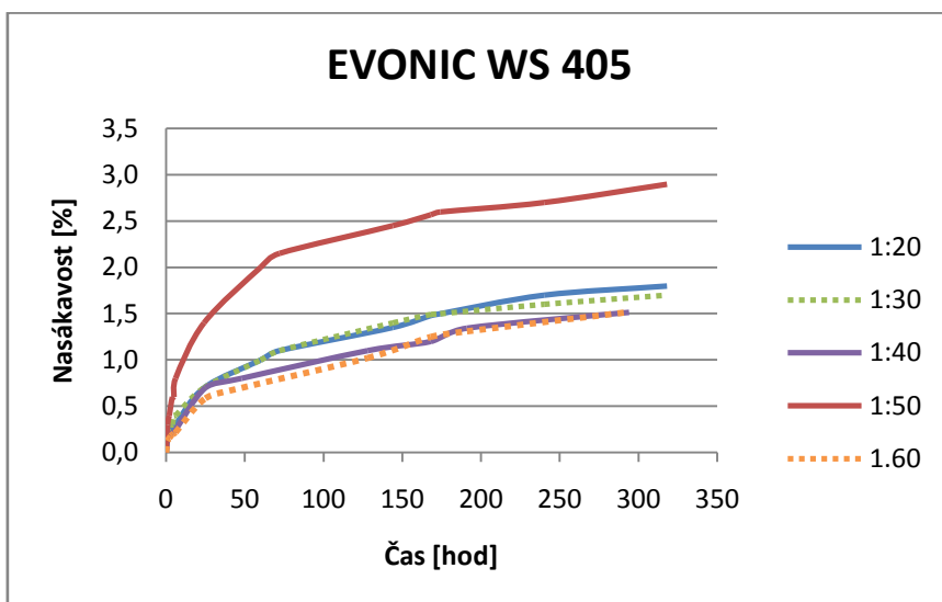
Graf 4 Závislost nasákavosti [%] na čase [h] ve zvolených koncentracích WS 405
