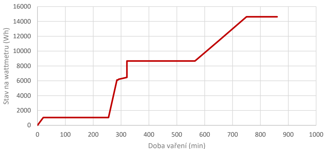
Obrázek 7-2 Spotřeba elektrické energie dekokčního způsobu vaření piva na ÚPI VUT v Brně
