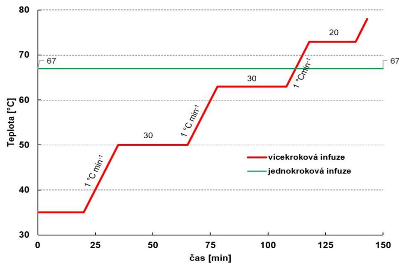
Obrázek 3-13 Průběh infuzního rmutování [39]
