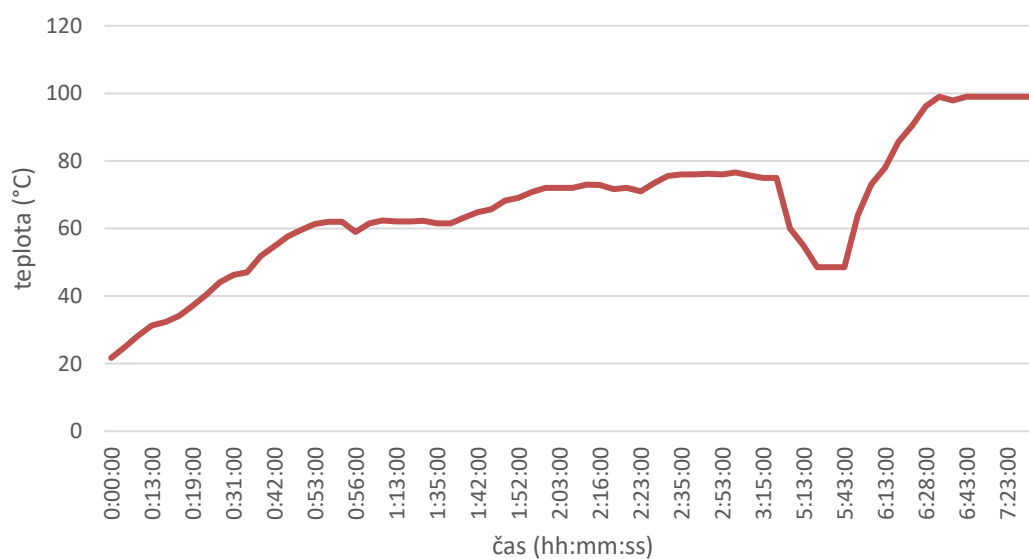
Obrázek 5-13 Skutečný teplotní průběh infuzního způsobu vaření piva
