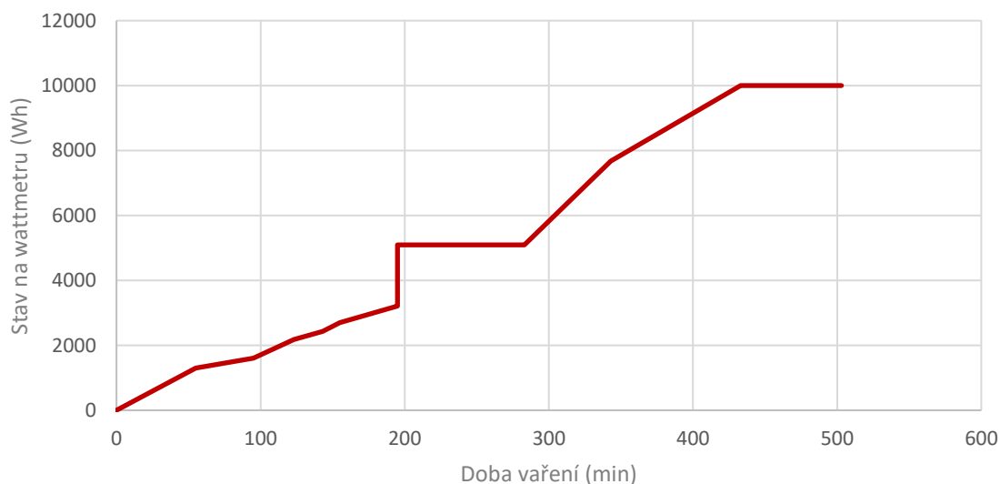
Obrázek 7-1 Spotřeba elektrické energie infuzního způsobu vaření piva na ÚPI VUT v Brně
