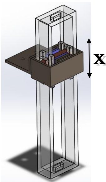
Obrázek 4- Elektromagnetický tlumič
