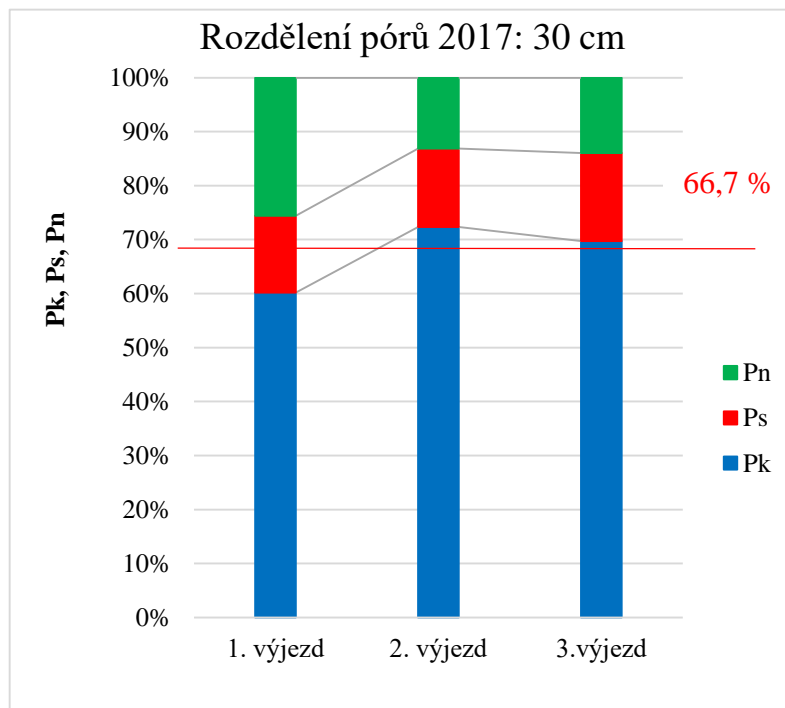
Obrázek 3.17 - Rozdělení pórů v podorníci v roce 2017
