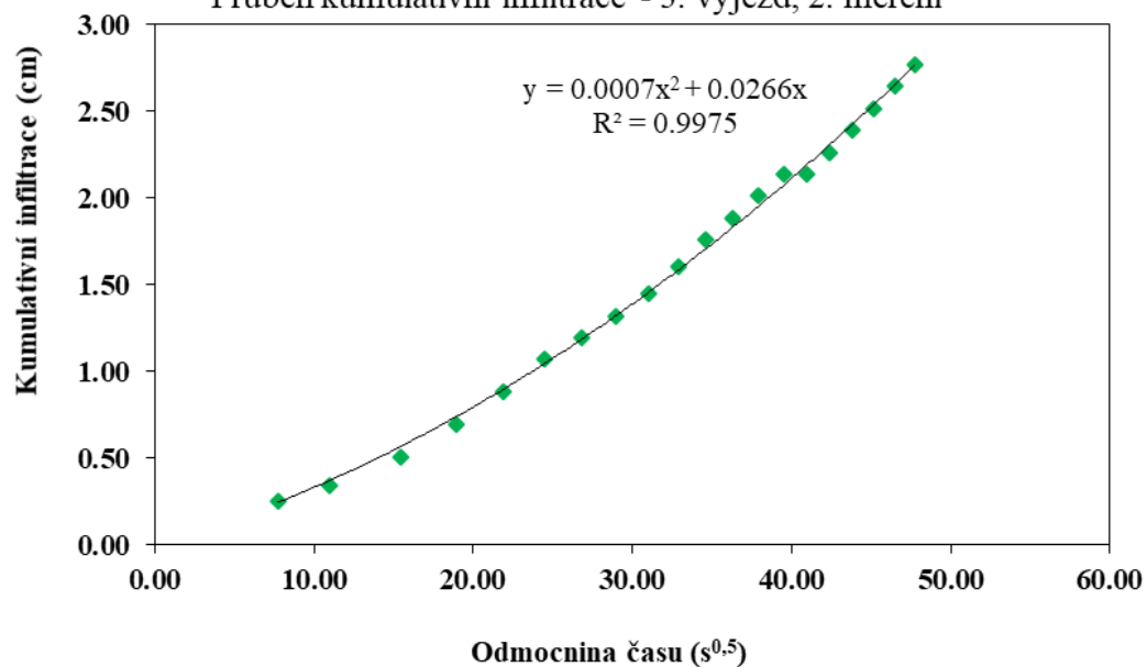
Průběh kumulativní infiltrace - 3. výjezd, 2. měření
