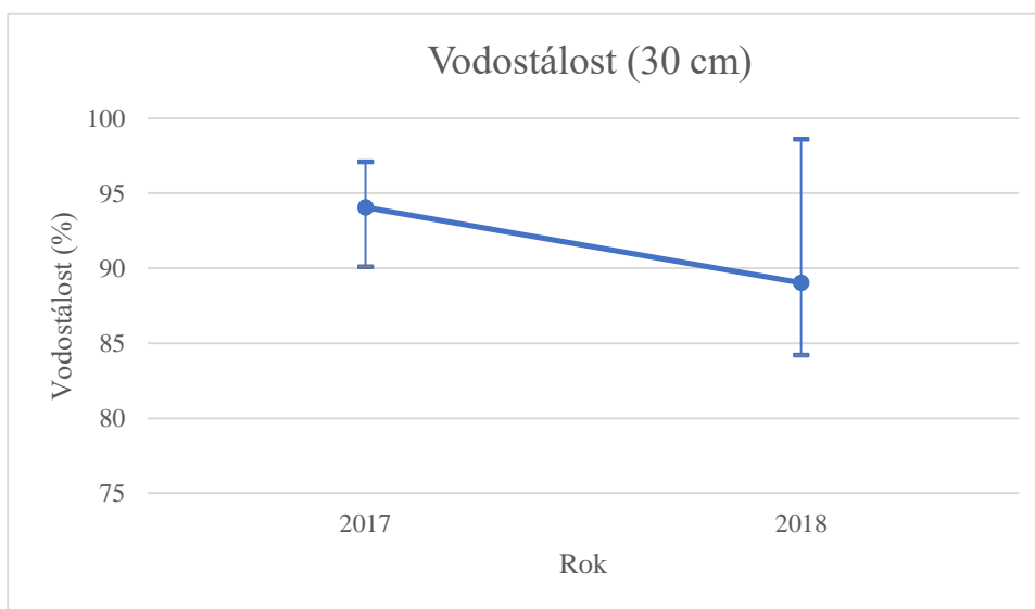
Obrázek 3.8 - Výsledky zkoušky vodostálosti podorníčí - minima, maxima a průměry
