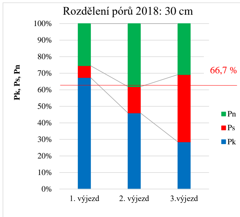
Obrázek 3.18 Rozdělení pórů v podorniči v roce 2018
