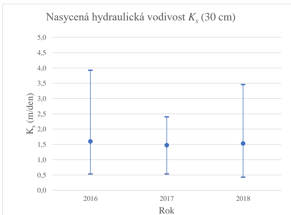
Obrázek 3.30 - Nasycená hydraulická vodivost K_s v hloubce 30 cm
