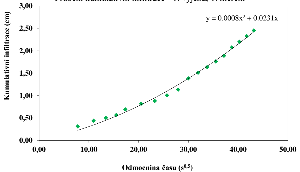
Průběh kumulativní infiltrace - 1. výjezd, 1. měření
