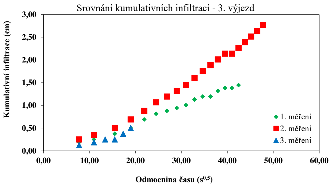
Obrázek 3.33 - Průběh kumulativní infiltrace – 3. Výjezd
